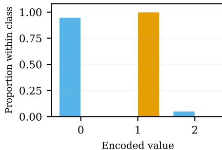
mqtt.msg (AUROC = 0.9482)
