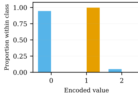
tcp.dstport (AUROC = 0.8350)
