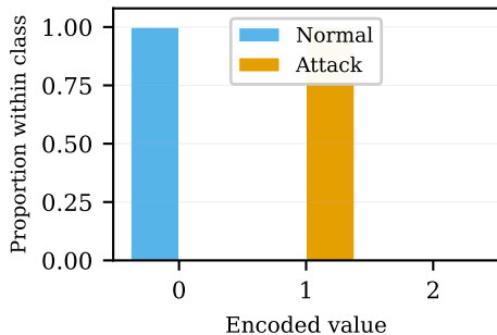
mqtt.protoname (AUROC = 0.9473)
