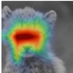
MaxViT-S
