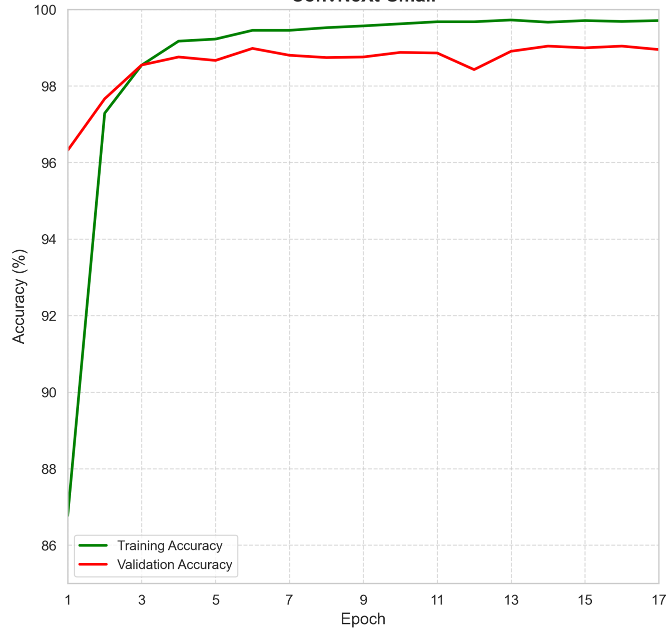
ConvNeXt-Small
