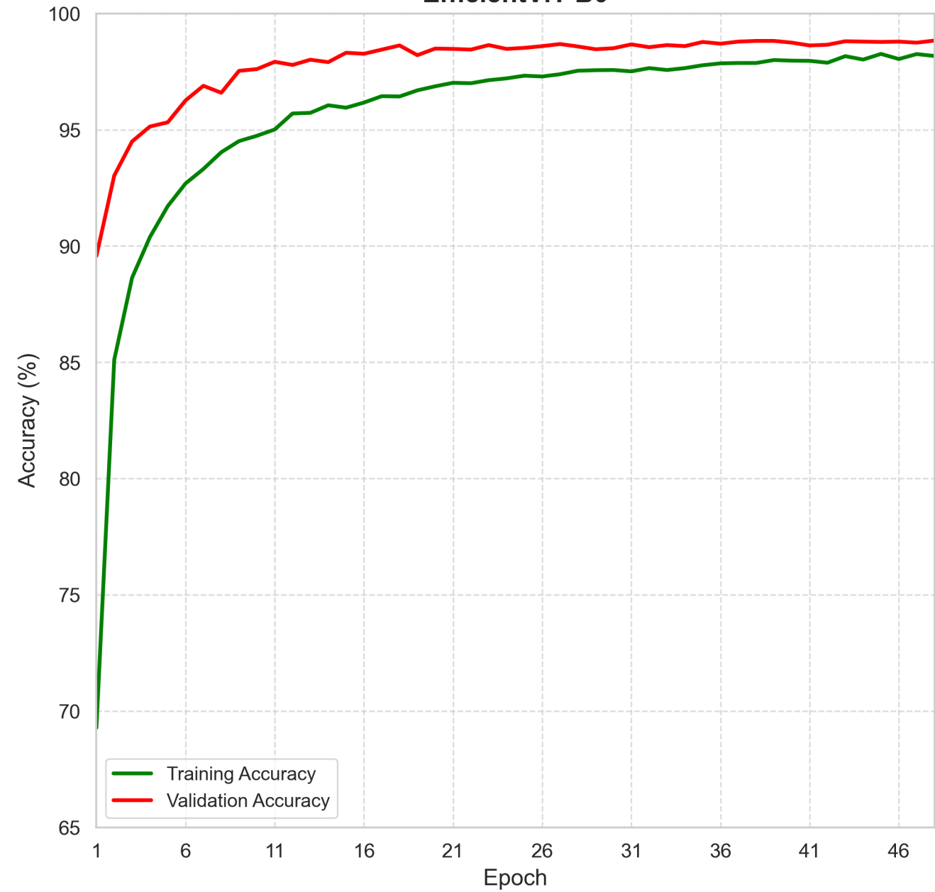
EfficientViT-B0
