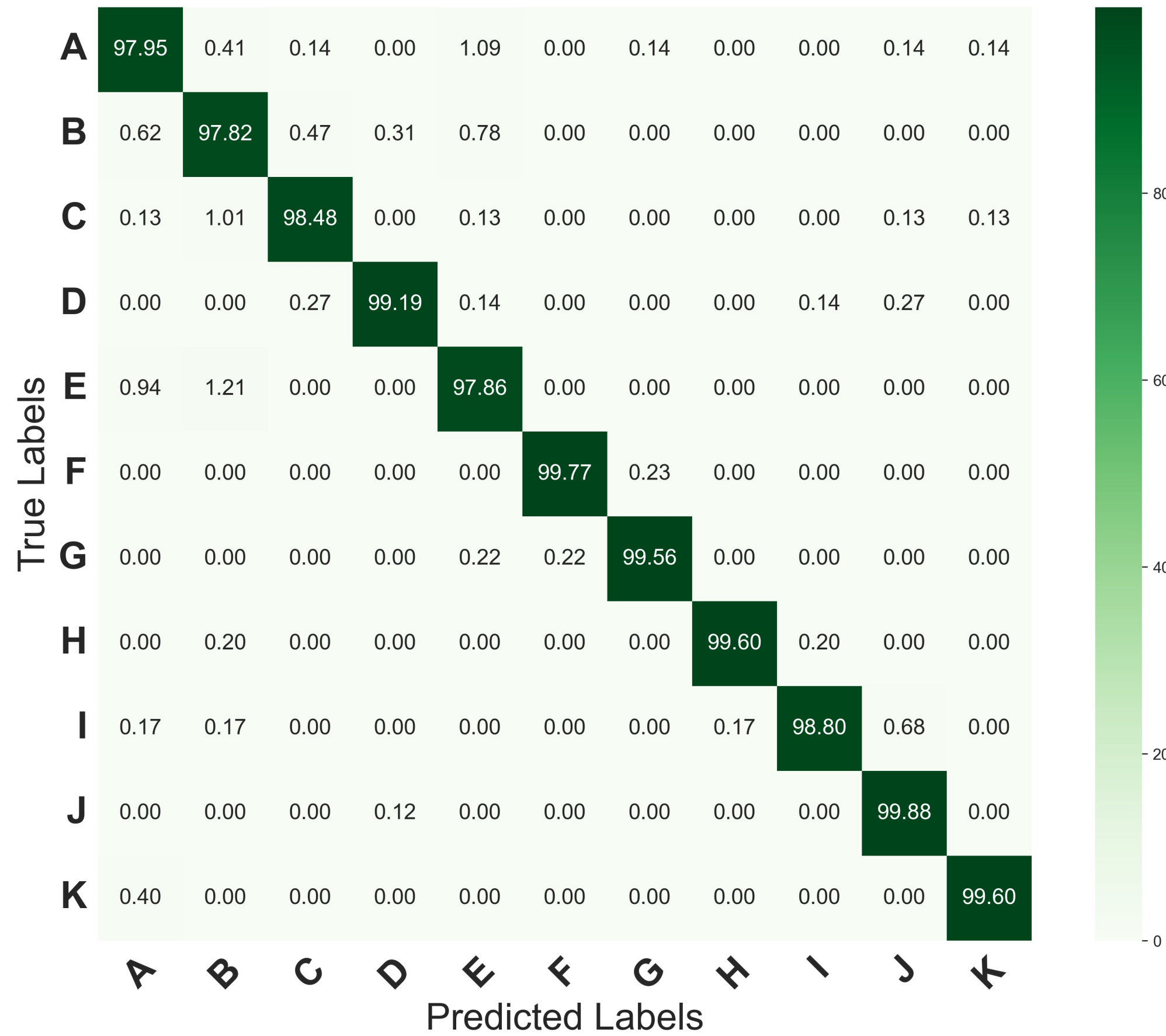
EfficientVit B0
