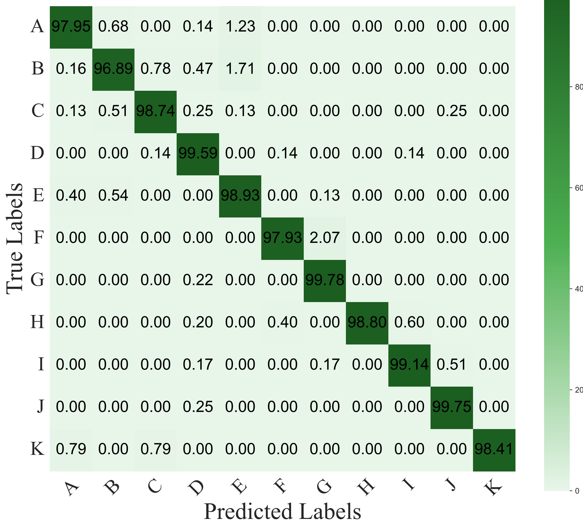
EfficientVit B0
