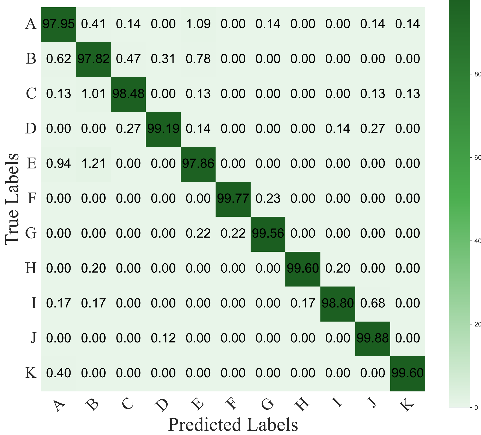
EfficientVit B0
