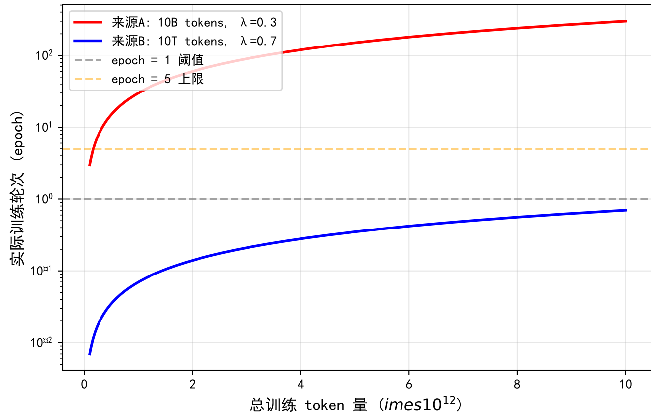
不同数据源的 epoch 随总训练量变化
