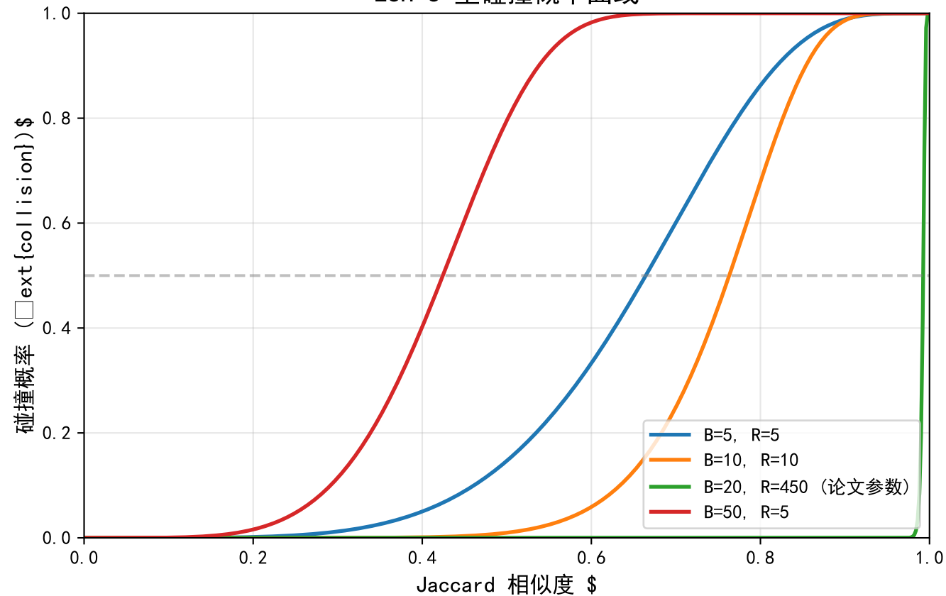
LSH S 型碰撞概率曲线
