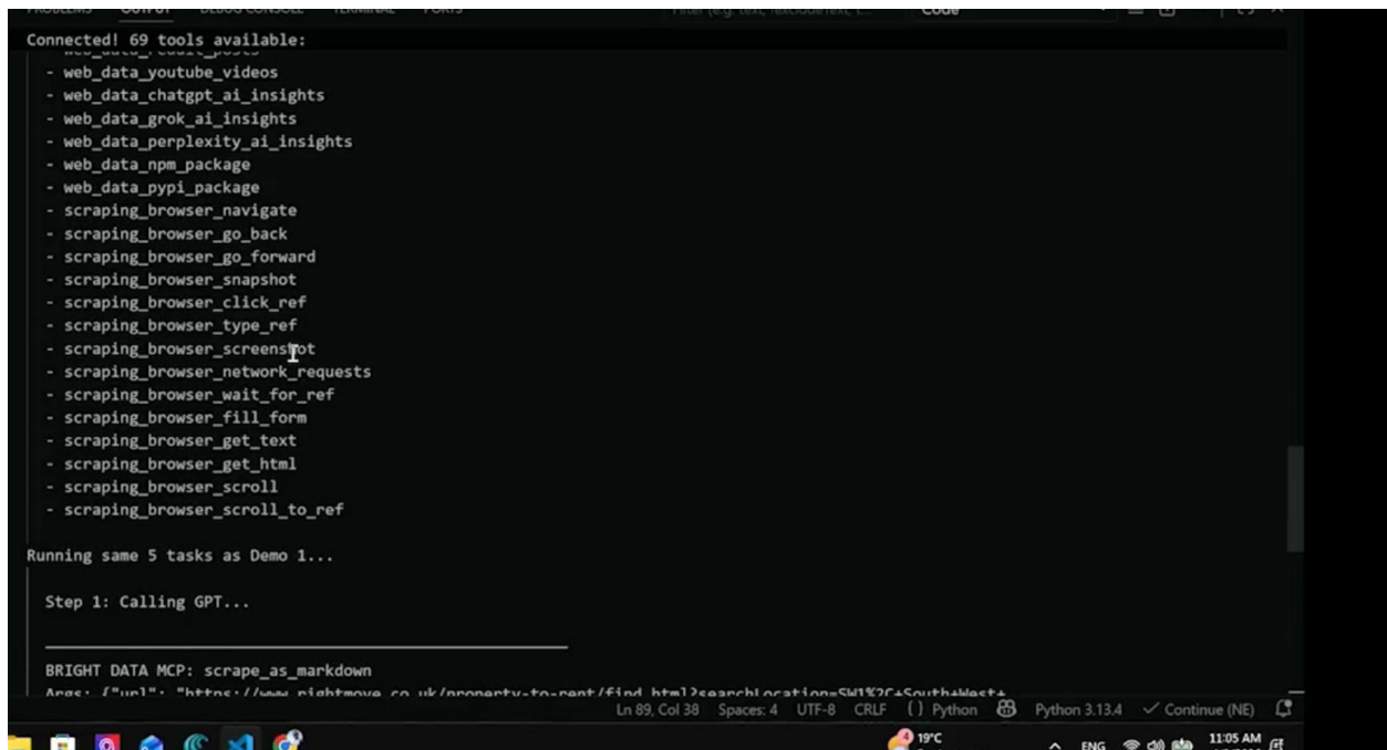
Figure 5: scraping_browser 工具族把远程浏览器暴露为可调用动作，包括导航、截图、点击、输入、表单填写与滚动。 9
