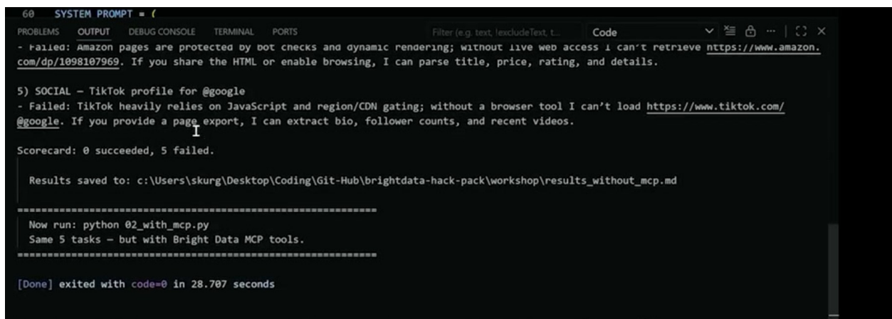
Figure 2: 无 MCP 基线的终端结果显示 Amazon 与 TikTok 等任务无法取得实时网页内容，最终计分为 0 成功、5 失败。 4
