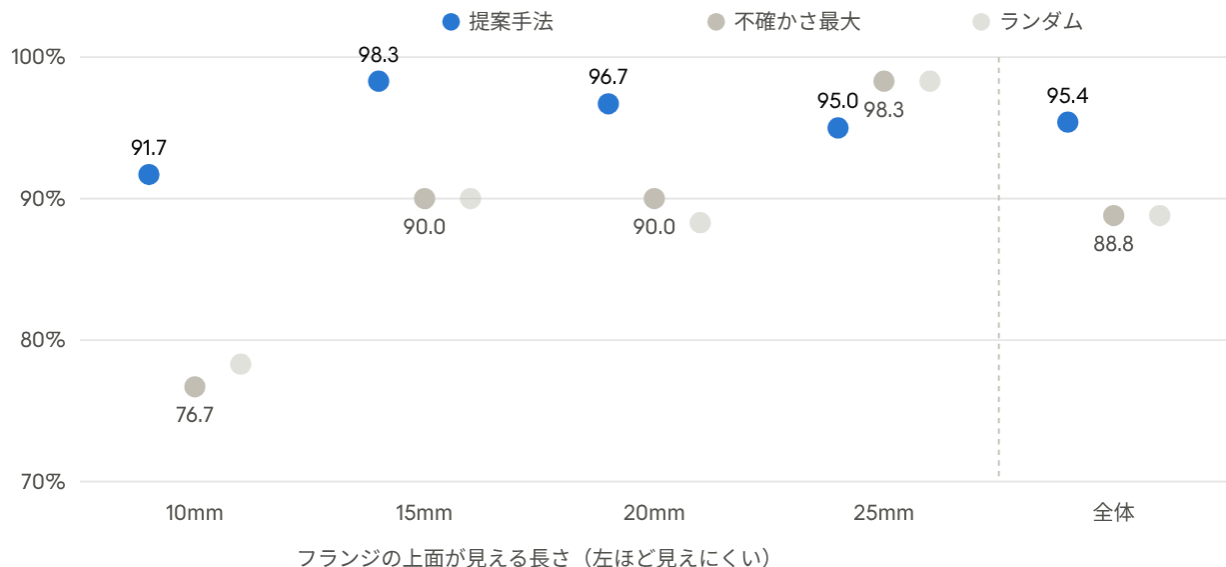
図2 run_touchsel.py の結果（240配置、触った後は天板の下のまま掴みに移る動き、2026年10月1日）
