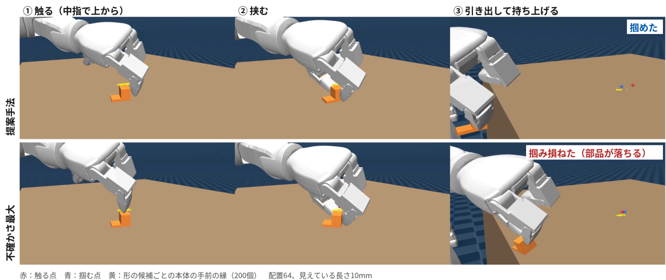
図3 配置64（見えている長さ10mm、本体は手前の面から15～31mm）。上段：提案手法は本体の奥の端より先（手前の面から43mm）を触って外れ、「本体はそこまで奥にない」と分かって本体の手前の縁の推定のばらつきが5.9mmから2.9mmに縮み、掴めた。下段：不確かさ最大は本体の真ん中（23mm）を触って当たったが、手前の縁のばらつきは4.3mm残り（予測した成功確率0.63）、掴み損ねた（view_trial.pyで撮影）。
