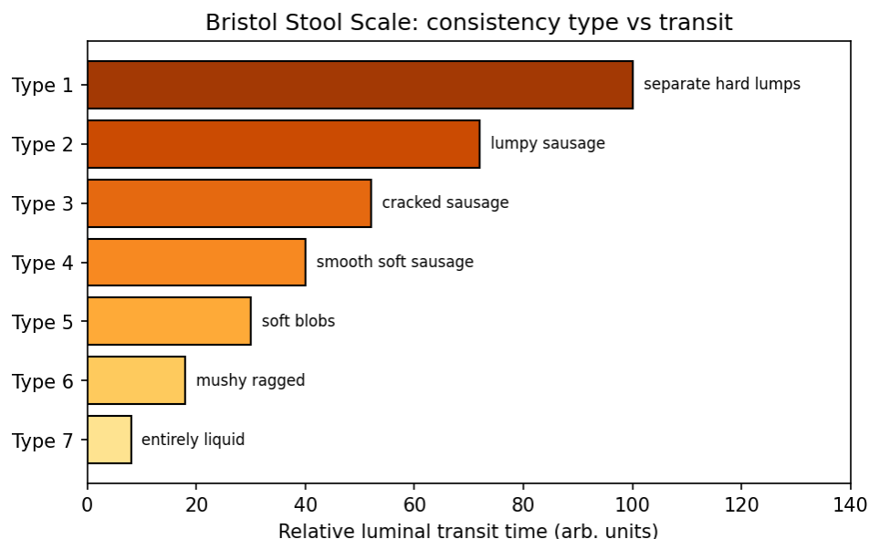
Figure 3: סולם הצואה של Bristol: טיפוס מרקם מול זמן מעבר.
