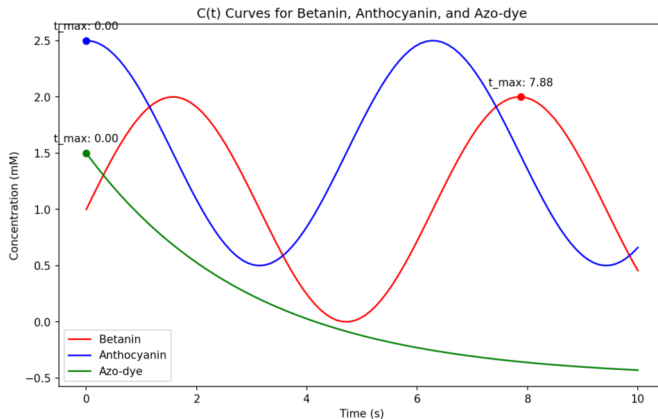
Figure 5: פרופילי ריכוז לומינלי C(t) עבור betanin מול anthocyanin מול צבע azo.
