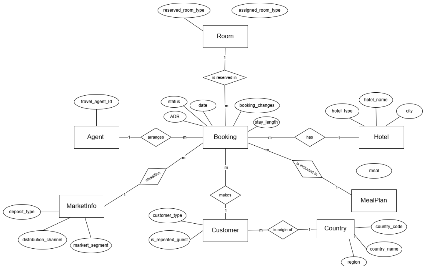
Figure 1 - ER Diagram
