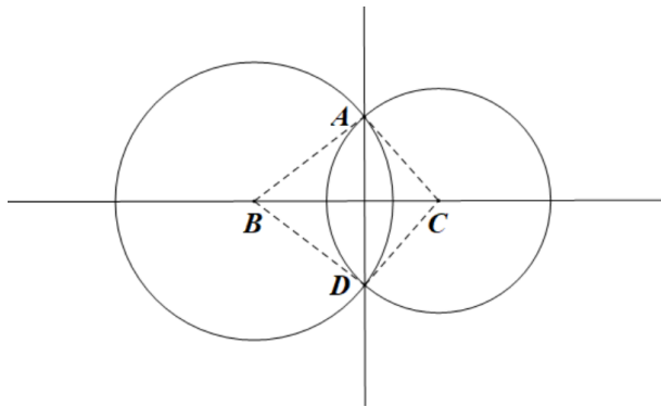
图 33.4: 尺规作过直线外一点的垂线
