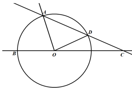
图 33.5: 有刻度直尺三等分角
