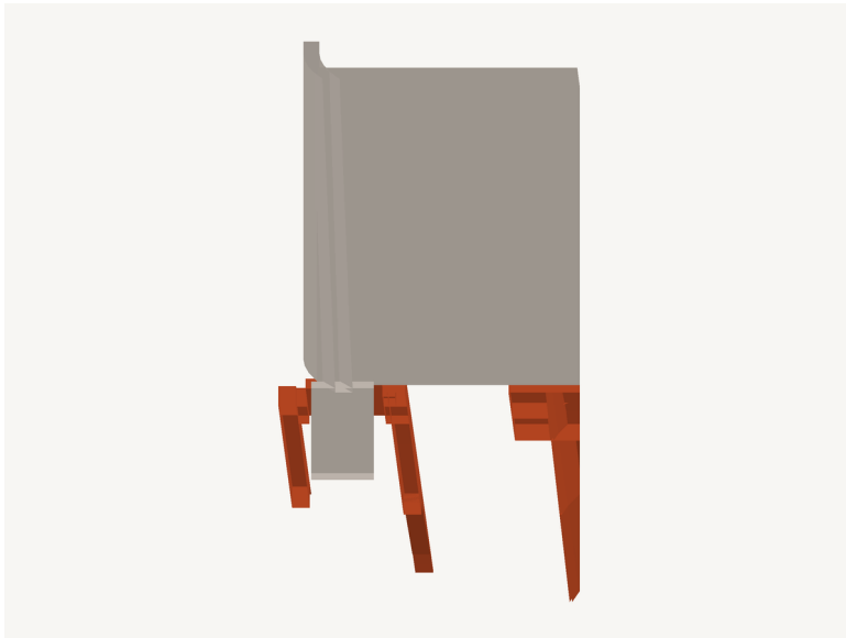
Corte: o pé do P (claro) pousado no aro do M; o pino dentro do bolsão
