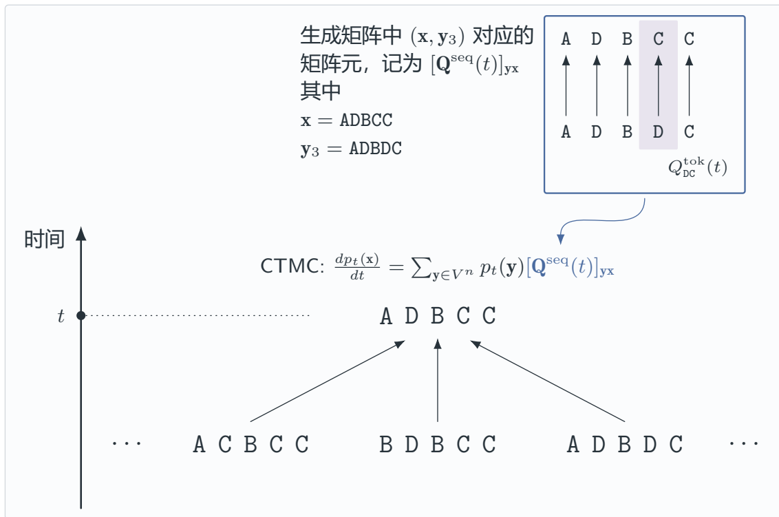
图 4.19: 连续时间马尔可夫链在 token 序列生成中的示意图。连续时间马尔可夫链在时间 t 的演化由 \frac{dp_t(\mathbf{x})}{dt} = \sum_{\mathbf{y} \in V^n} p_t(\mathbf{y}) [\mathbf{Q}^{\text{seq}}(t)]_{\mathbf{y}\mathbf{x}} 描述。该方程表明, 目标序列 \mathbf{x} (例如 ADBCC) 的概率随时间的变化, 由所有可能源序列 (例如 \mathbf{y}_1 、 \mathbf{y}_2 、 \mathbf{y}_3 ) 共同决定, 其中每个源序列的贡献由其当前概率与对应的序列级转移速率 [\mathbf{Q}^{\text{seq}}(t)]_{\mathbf{y}\mathbf{x}} 共同确定。序列级转移速率进一步由底层的 token 级动力学决定。例如, 从序列 \mathbf{y}_3 到 \mathbf{x} 的转移仅涉及单个 token 的变化, 即第四个 token 从 D 变为 C, 其对应速率为 Q_{\text{DC}}^{\text{tok}}(t) 。需要注意的是, 虽然连续时间马尔可夫链在连续时间中描述系统动力学, 但状态之间的转移仍以离散跳跃的形式发生, 而非连续变化。
