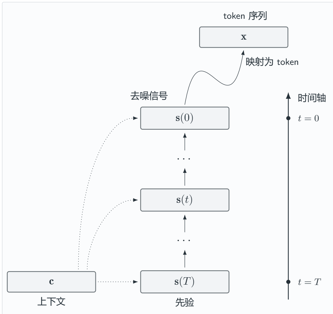
图 4.17: 基于扩散模型的非自回归生成示意图。生成过程被建模为状态 s(t) 随时间 t 的演化过程。其中 s(T) 表示起始点（先验分布）， s(0) 表示终点（完全去噪信号）。上下文信息 c 在生成过程中被注入状态变量。最终输出是从 s(0) 映射得到的 token 序列。
