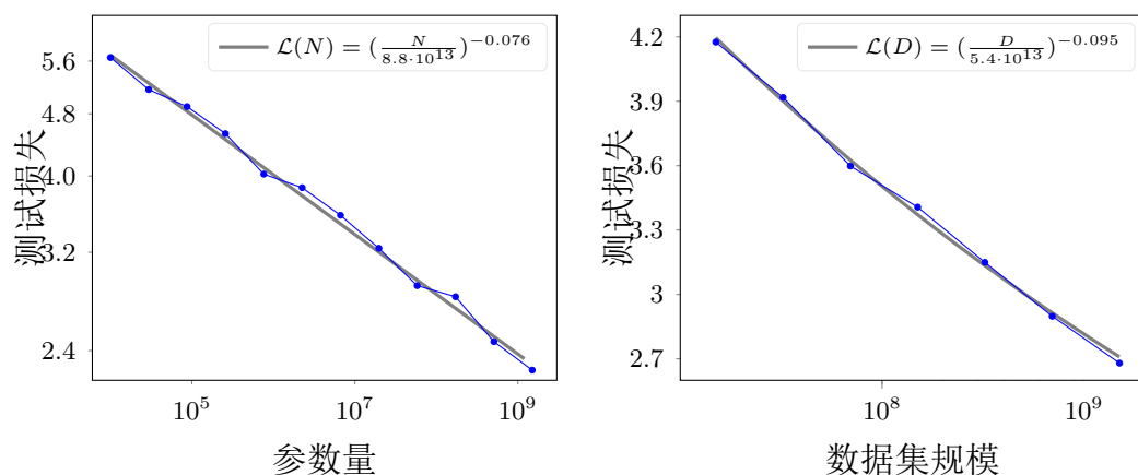
图 3.2: 测试损失与模型参数量 N 及训练数据量 D 的关系。左: \mathcal{L}(N) = \left(\frac{N}{8.8 \times 10^{13}}\right)^{-0.076} ; 右: \mathcal{L}(D) = \left(\frac{D}{5.4 \times 10^{13}}\right)^{-0.095} 。均基于 [136] 报告的拟合结果。
