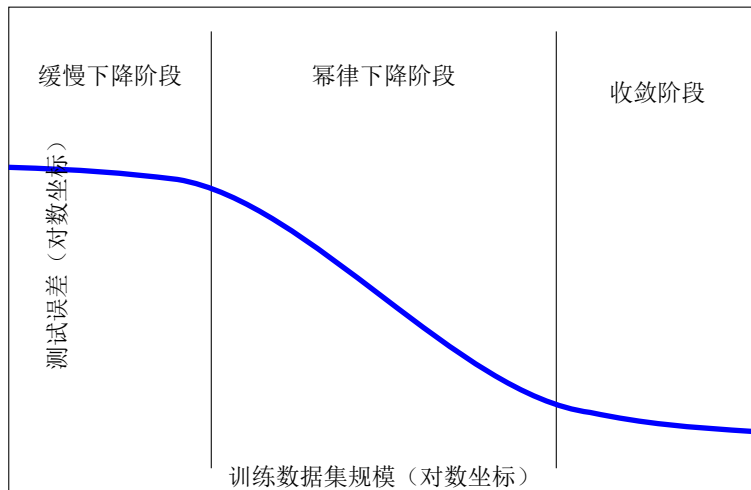
图 3.3: 测试误差随训练数据量变化的缩放曲线 [124]。在大多数实用区间内，误差按幂律衰减；当数据量极大时衰减趋缓，但误差始终存在一个大于零的下界（不可约误差）。
