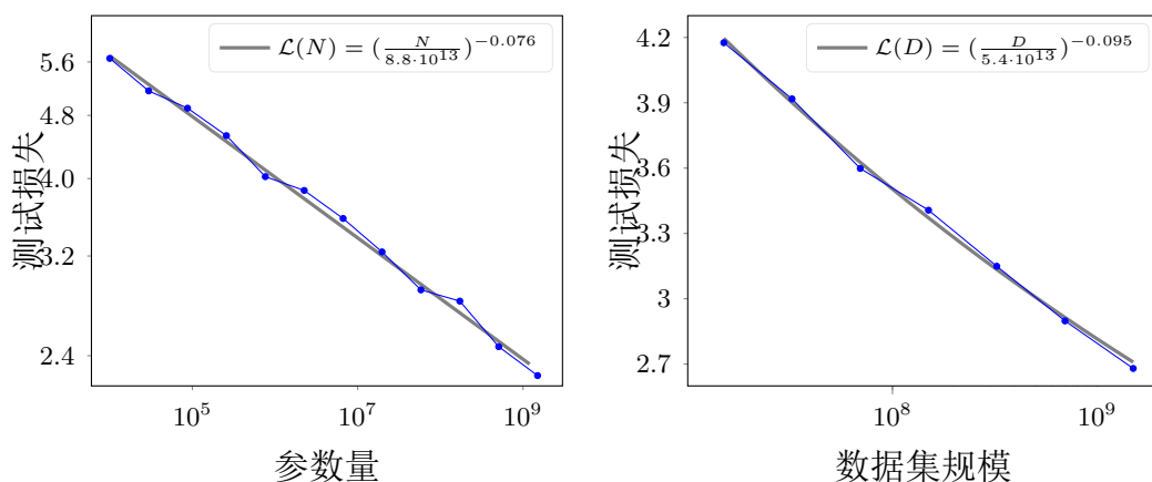
图 3.2: 测试损失与模型参数量 N 及训练数据量 D 的关系。左: \mathcal{L}(N) = \left(\frac{N}{8.8 \times 10^{13}}\right)^{-0.076} ; 右: \mathcal{L}(D) = \left(\frac{D}{5.4 \times 10^{13}}\right)^{-0.095} 。均基于 [139] 报告的拟合结果。
