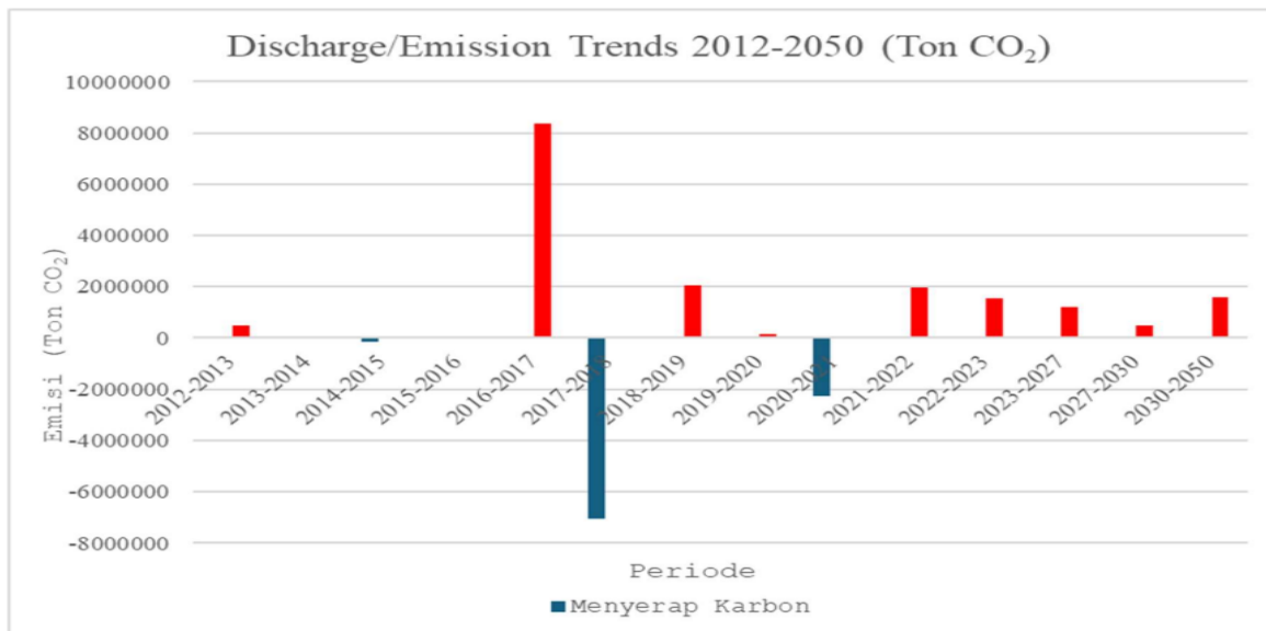
Gambar 2.13 Tren Debit/Emisi Kabupaten Aceh Tengah Tahun 2012-2050 (Ton CO 2 )
