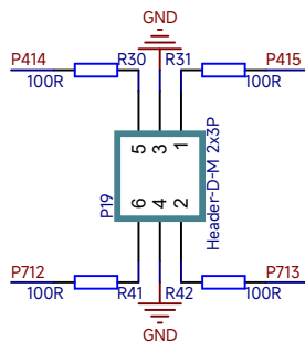
有刷电机信号接口
