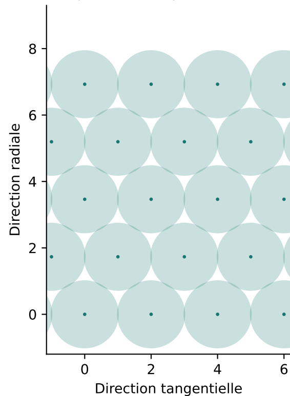
Période 2 : alternance Espacement moyen : 1.732051
