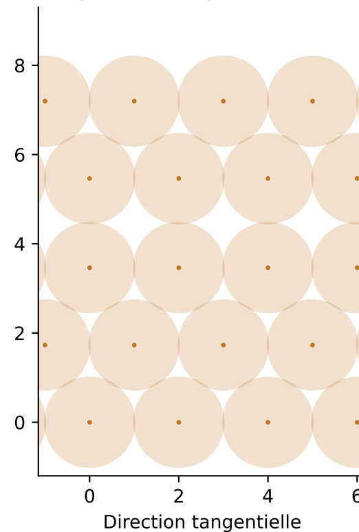
Période 3 : un défaut Espacement moyen : 1.821367
