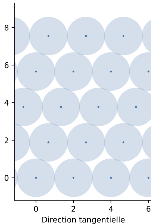
Période 3 : pas uniforme Espacement moyen : 1.885618
