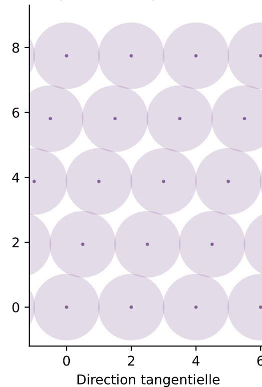
Vraie période 4 : quarts de pas Espacement moyen : 1.936492
