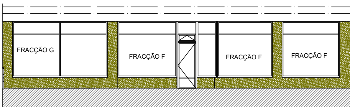
ALÇADO POSTERIOR
