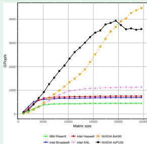
Figure 3 – Etude de la portabilité des performances de l'application X sur l'ensemble des architectures testées.
