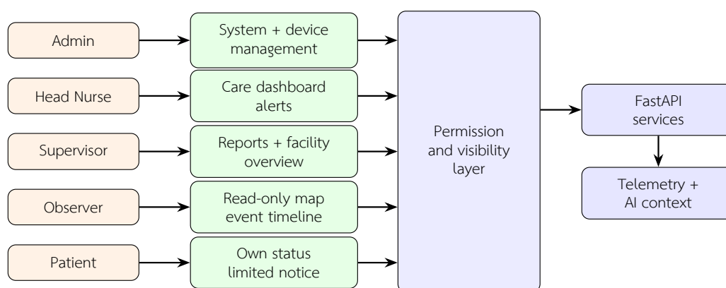
รูปที่ 3.13: HMI role flow ของระบบ WheelSense แสดงความสัมพันธ์ระหว่างบทบาทผู้ใช้ หน้าจอ และ service ที่เกี่ยวข้อง
