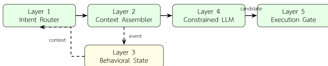
รูปที่ 3.17: โครงสร้าง AI pipeline 5 layer โดย Layer 3 ทำหน้าที่เตรียม behavioral context นอกเส้นทาง execute หลัก
