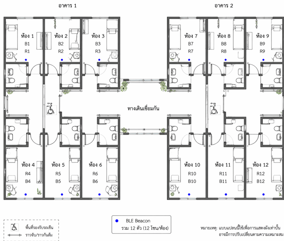
รูปที่ 3.9: แผนผังพื้นที่ทดลองที่ใช้วาง BLE node สำหรับเก็บค่า RSSI ภายในอาคาร
