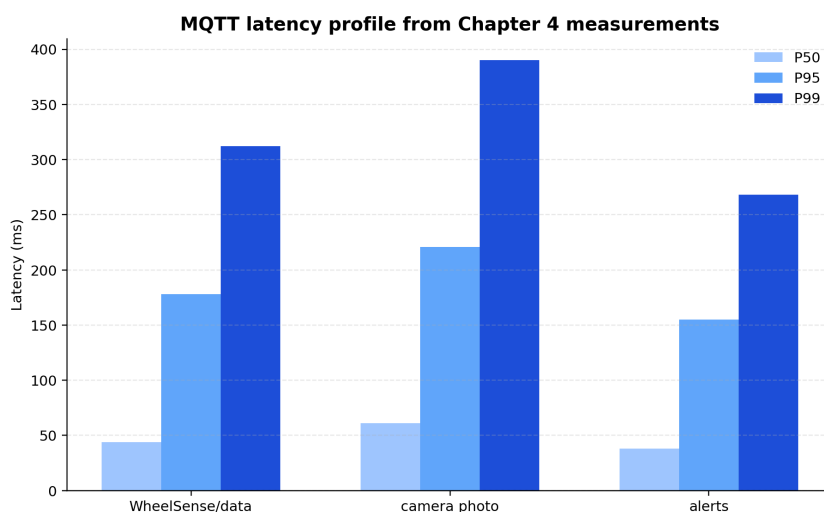
รูปที่ 4.5: กราฟสรุปการกระจายของ latency ในเส้นทาง MQTT ระหว่างการทดสอบ
