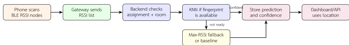
รูปที่ 3.10: Flowchart การส่งข้อมูล RSSI และการประเมินตำแหน่งด้วย KNN หรือ max-RSSI fallback
