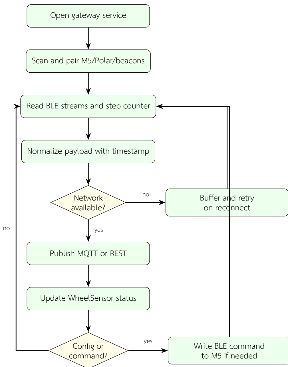
รูปที่ 3.7: วงรอบการทำงานของ Flutter mobile gateway สำหรับรวมข้อมูล Polar, M5StickC Plus2, RSSI และ step counter
