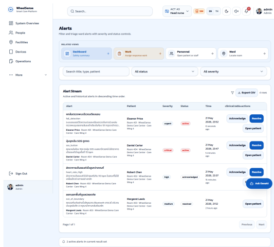
(a) หน้า Alerts ของ Head Nurse
