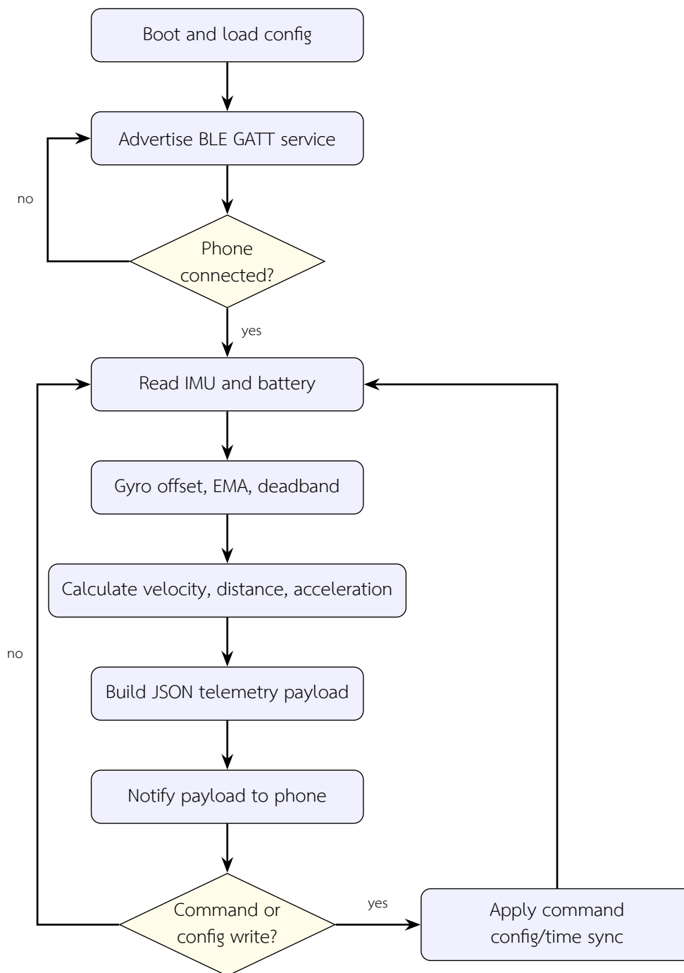
รูปที่ 3.5: แผนผังวงจรการทำงานของเฟิร์มแวร์ M5StickC Plus2 แบบ BLE wheelchair sensor
