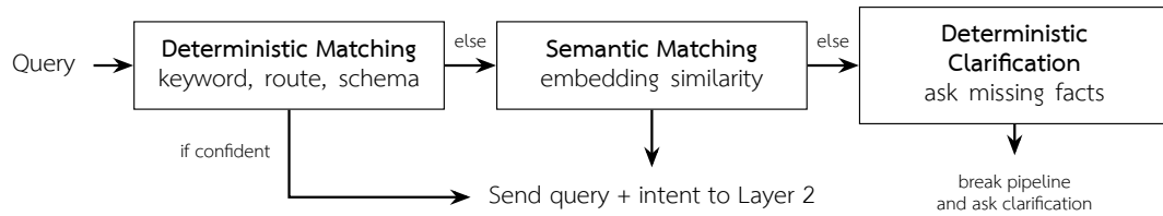
รูปที่ 3.18: Layer 1 Intent Router สำหรับจับเจตนาแบบ deterministic ก่อนใช้ semantic matching และ clarification
