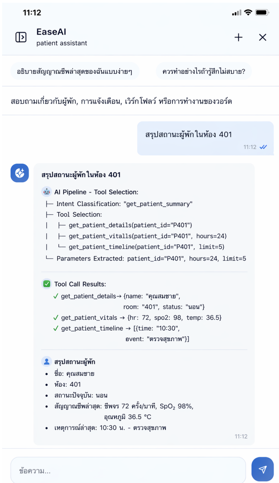
รูปที่ 4.8: ตัวอย่างการเลือกเครื่องมือโดย AI เพื่อตอบคำถาม
