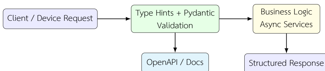
รูปที่ 2.13: กระบวนการทำงานของ FastAPI ที่เชื่อมการตรวจสอบข้อมูลเข้ากับเอกสาร API อัตโนมัติ
