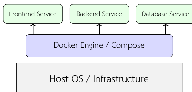
รูปที่ 2.18: การจัดวางบริการหลักของระบบในสภาพแวดล้อมคอนเทนเนอร์
