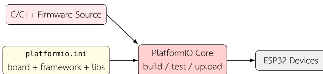
รูปที่ 2.22: กระบวนการพัฒนาและติดตั้งเฟิร์มแวร์ผ่าน PlatformIO
