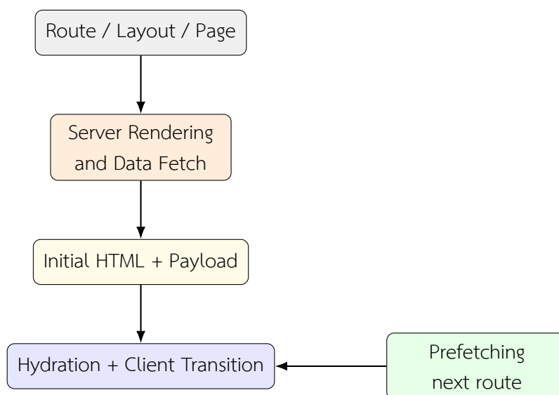
รูปที่ 2.15: แนวคิดการเรนเดอร์และการนำทางของ Next.js สำหรับเว็บแอปพลิเคชันเชิงปฏิบัติการ
