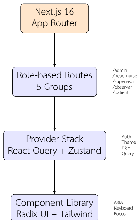
รูปที่ 3.15: สถาปัตยกรรมแดชบอร์ดเว็บ
