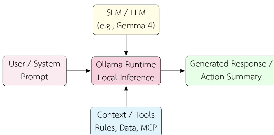
รูปที่ 2.19: แนวคิดการให้บริการโมเดลภาษาขนาดใหญ่ภายในระบบผ่าน Ollama
