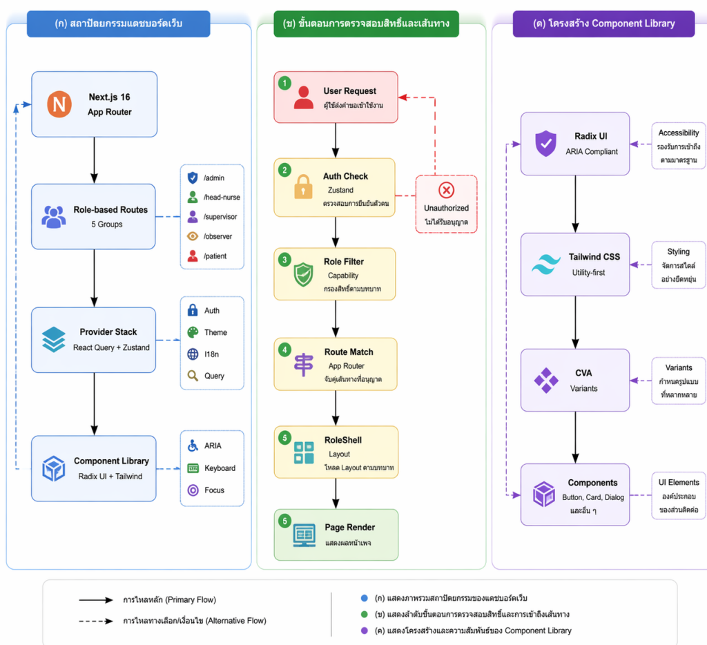
รูปที่ 3.16: ขั้นตอนการตรวจสอบสิทธิ์และโครงสร้าง Component Library
