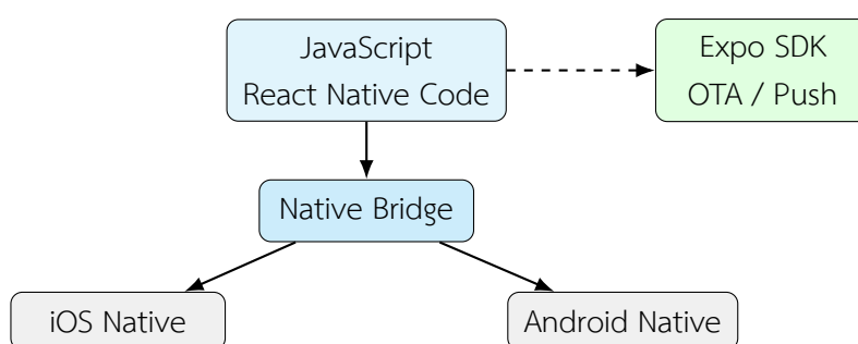
รูปที่ 2.16: สถาปัตยกรรมการทำงานของ React Native ผ่าน Native Bridge และการเสริมความสามารถด้วย Expo
