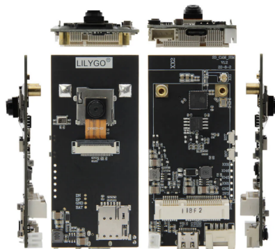
รูปที่ 2.9: ลักษณะภายนอกของโหนดกล้อง Lilygo T-SimCam ที่รองรับการประมวลผลภาพเบื้องต้น
