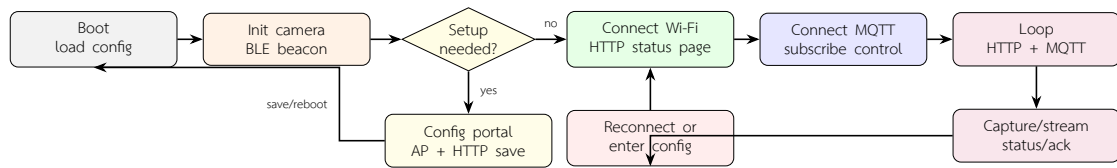
รูปที่ 3.3: วงรอบเฟิร์มแวร์ Node T-SimCam สำหรับ config portal, HTTP status, MQTT control และการส่งภาพ
