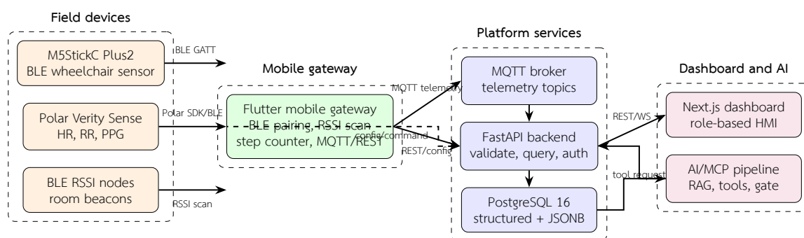
รูปที่ 3.1: สถาปัตยกรรมโดยรวมของระบบ WheelSense จากอุปกรณ์ภาคสนามไปยัง mobile gateway, platform services, dashboard และ AI
