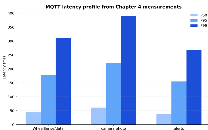
รูปที่ 4.6: กราฟสรุปการกระจายของ latency ในเส้นทาง MQTT ระหว่างการทดสอบ
