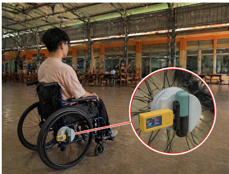
รูปที่ 4.1: การติดตั้ง M5StickC Plus2 บนรถเข็นสำหรับทดสอบข้อมูล IMU และ telemetry
