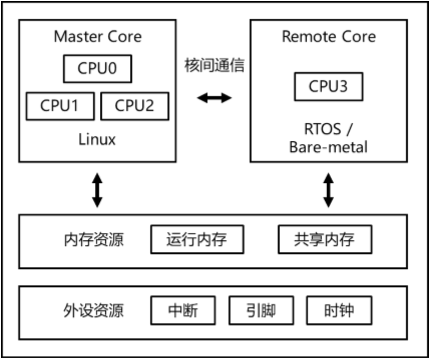
图 4-1-1 Linux + RTOS / Bare-metal 系统架构
