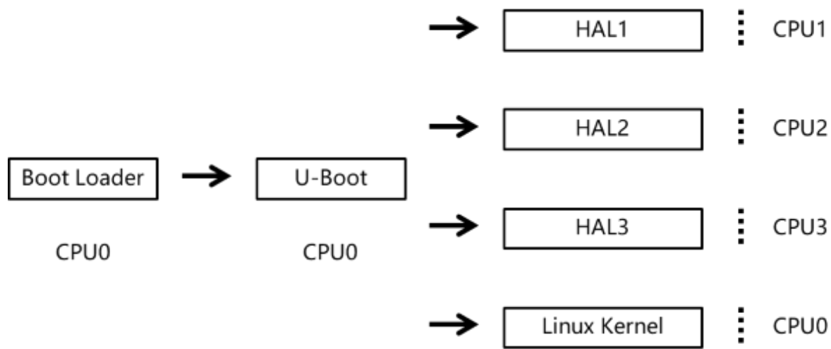
图 5-1-3 kernel + 3 * hal
