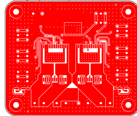
Top Layer (Scale 1:1)
