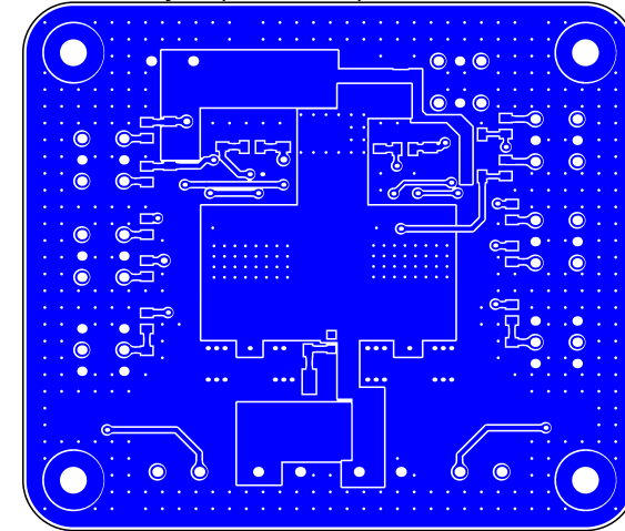
Bottom Layer (Scale 1:1)
