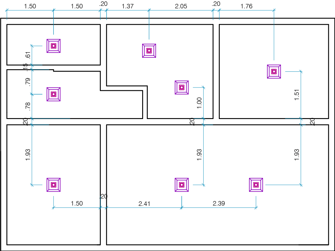
PLANTA BAIXA PONTOS LUMINICOS____1/75
