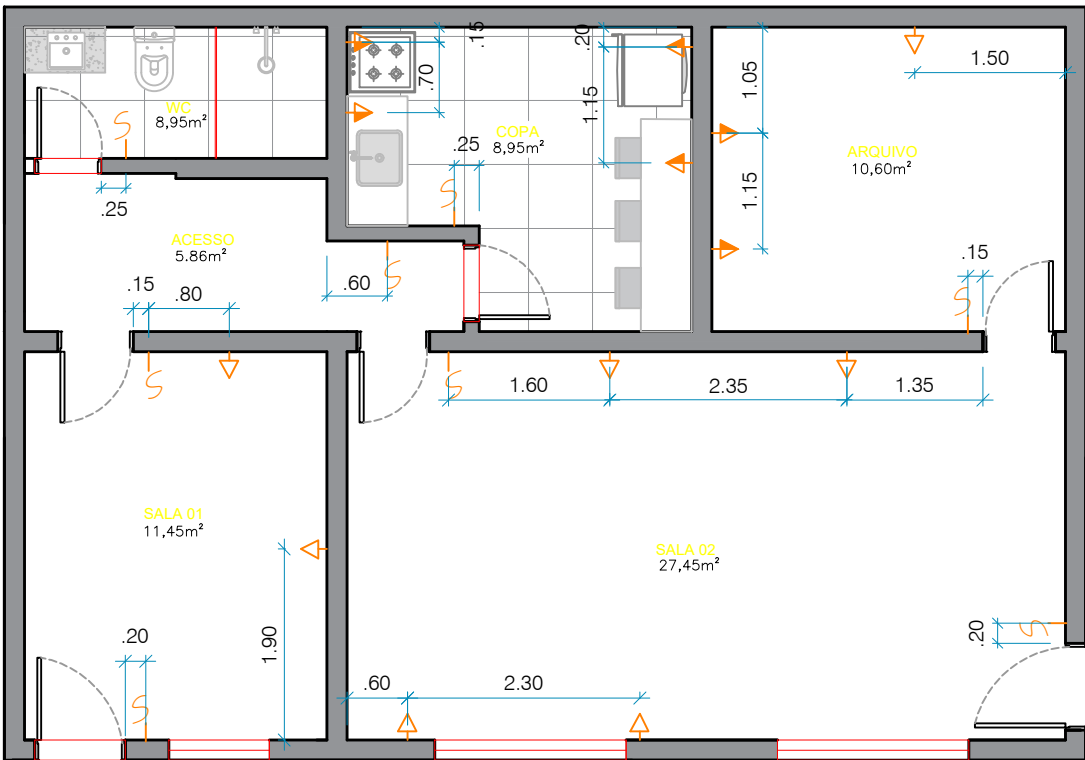
PLANTA BAIXA PONTOS ELETRICOS____1/75
