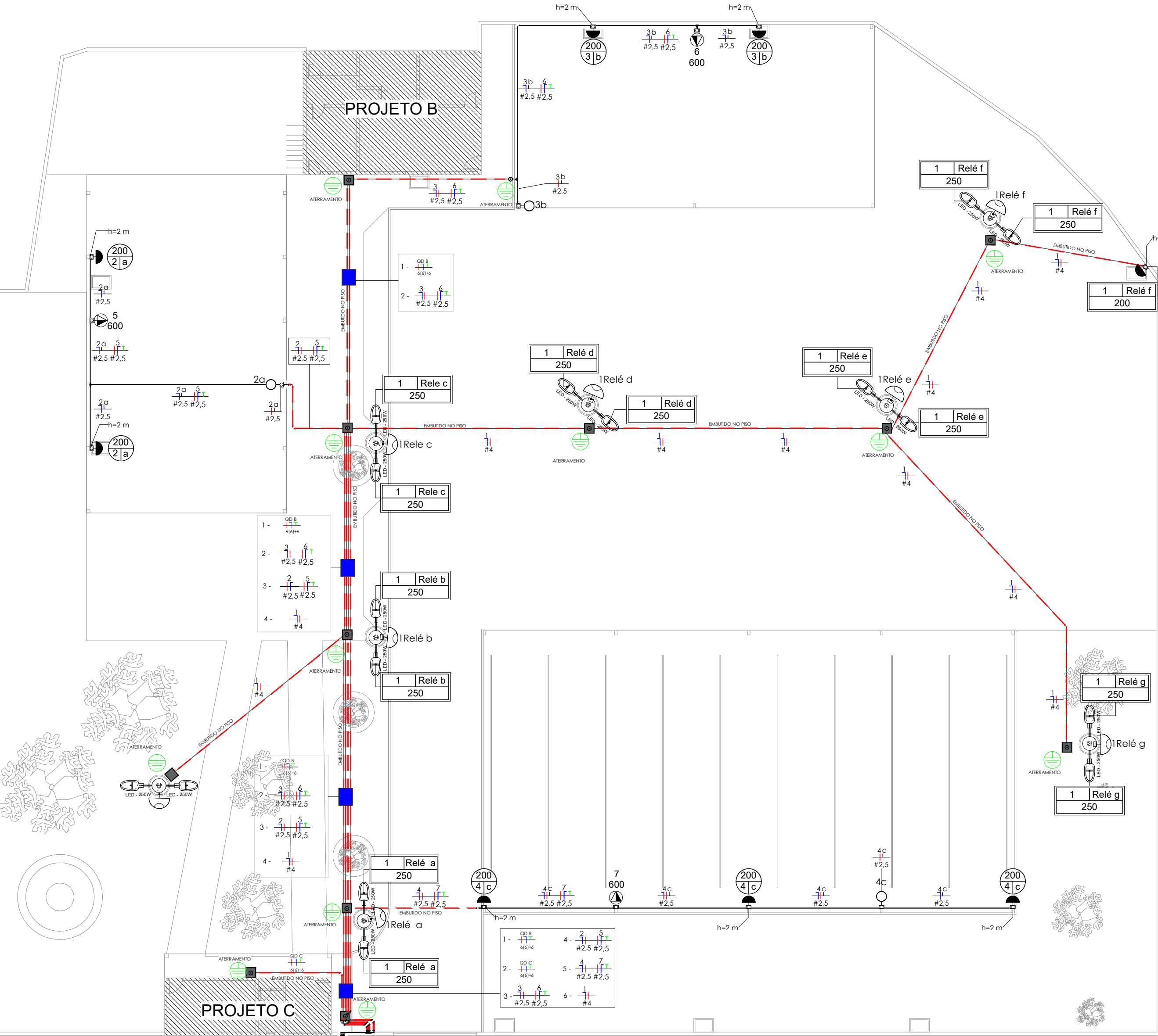
PLANTA BAIXA - PLANTA GERAL
