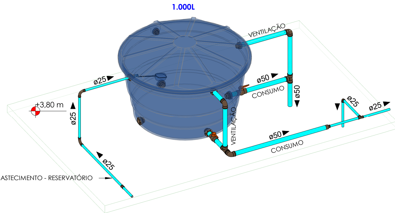
ISOMÉTRICA 05 - CAIXA D'ÁGUA - ESC 1/25
