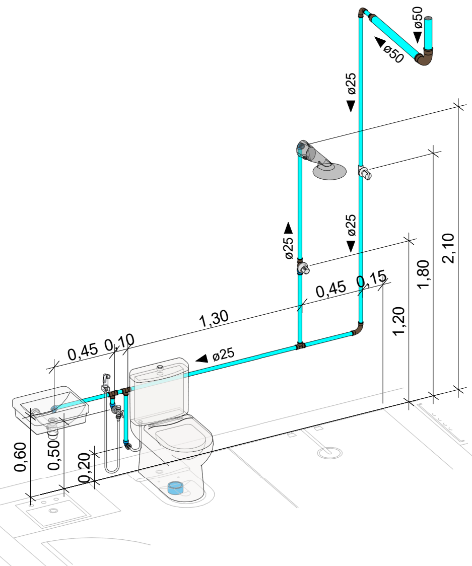
ISOMÉTRICA 03 - WC - ESC 1/25
