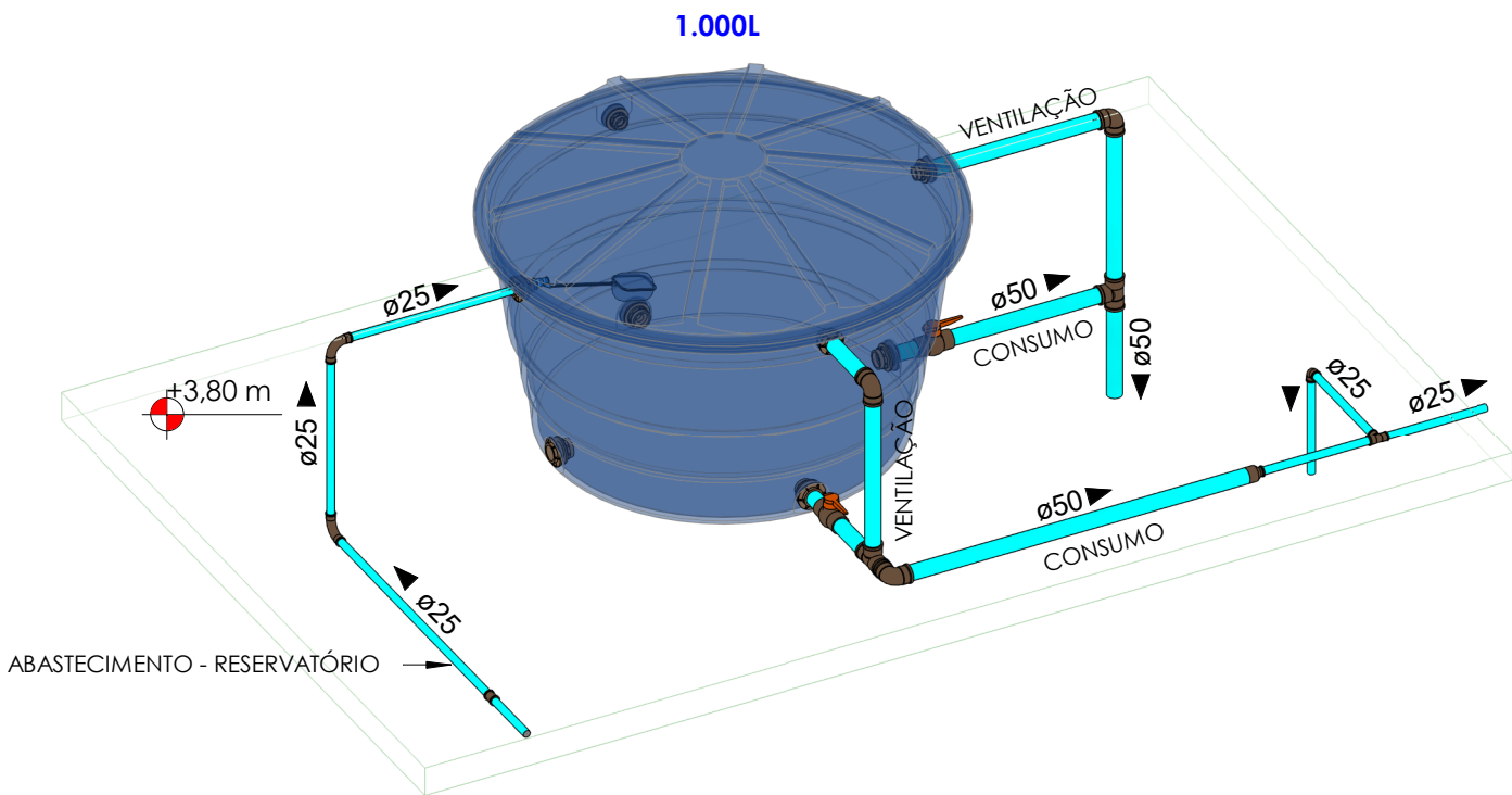
ISOMÉTRICA 05 - CAIXA D'ÁGUA - ESC 1/25
