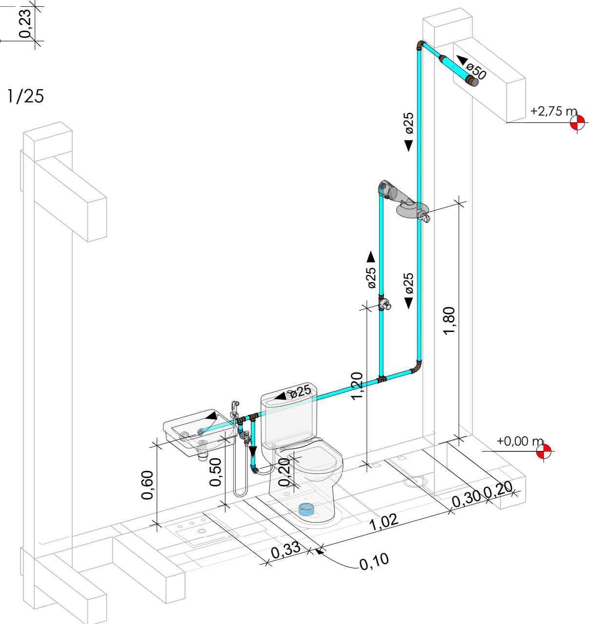
ISOMÉTRICA 01 - WC 1 - ESC 1/25
