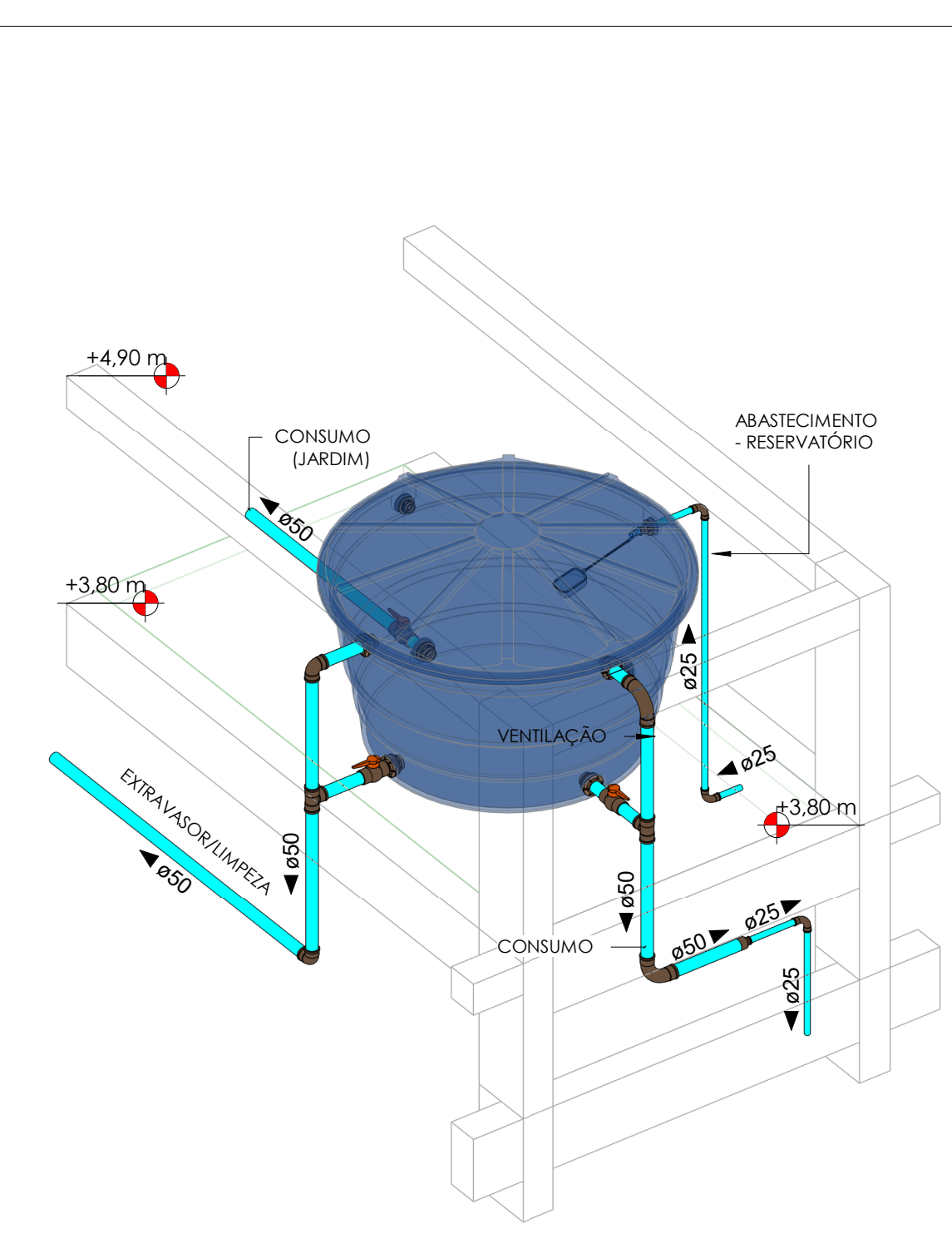
ISOMÉTRICA 02 - WC 2 - ESC 1/25
