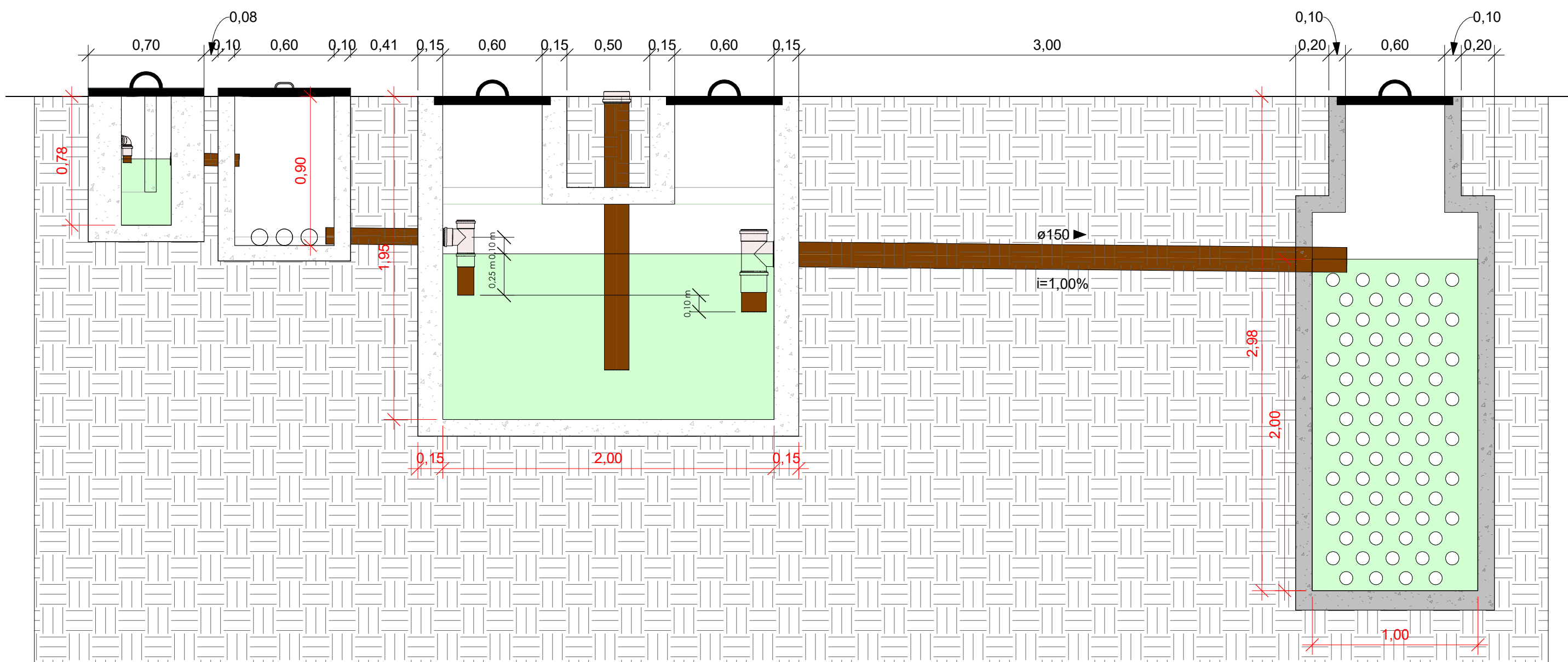
CORTE CC
