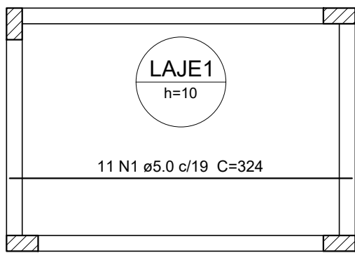
Armação positiva das lajes do pavimento +275 (Eixo X) escala 1:50
