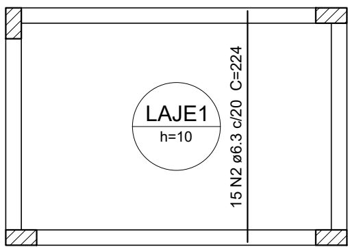
Armação positiva das lajes do pavimento +275 (Eixo Y) escala 1:50
