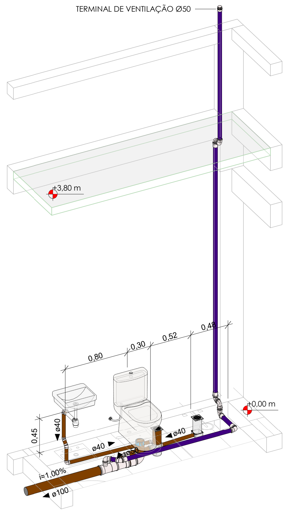
ISOMÉTRICA 02 - WC_MONITORAMENTO - ESC
