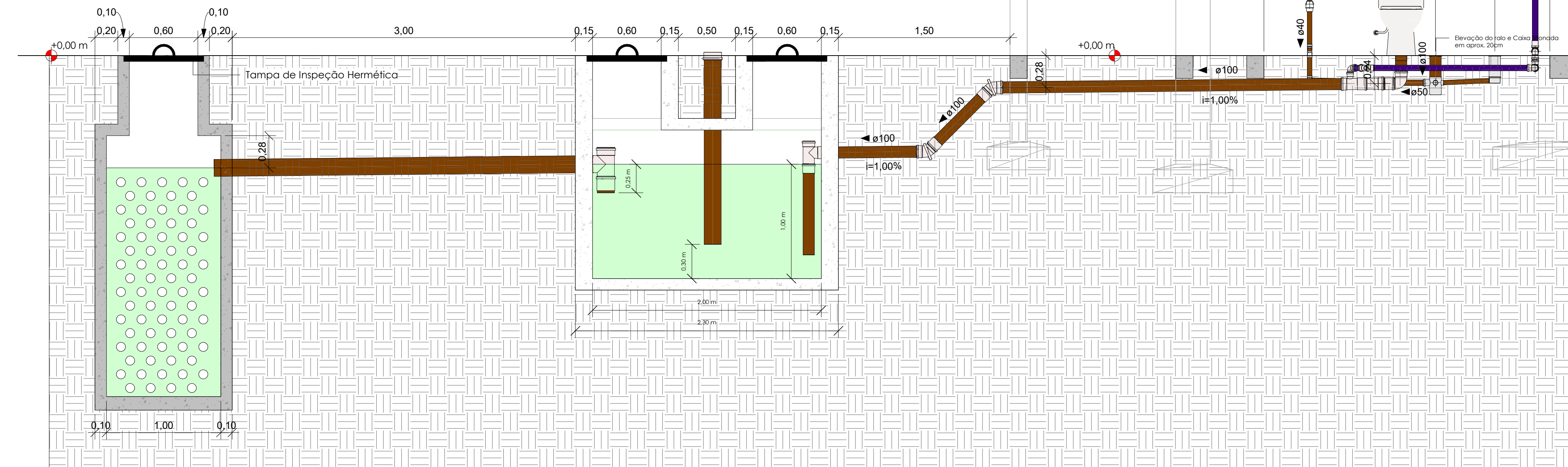
CORTE AA
