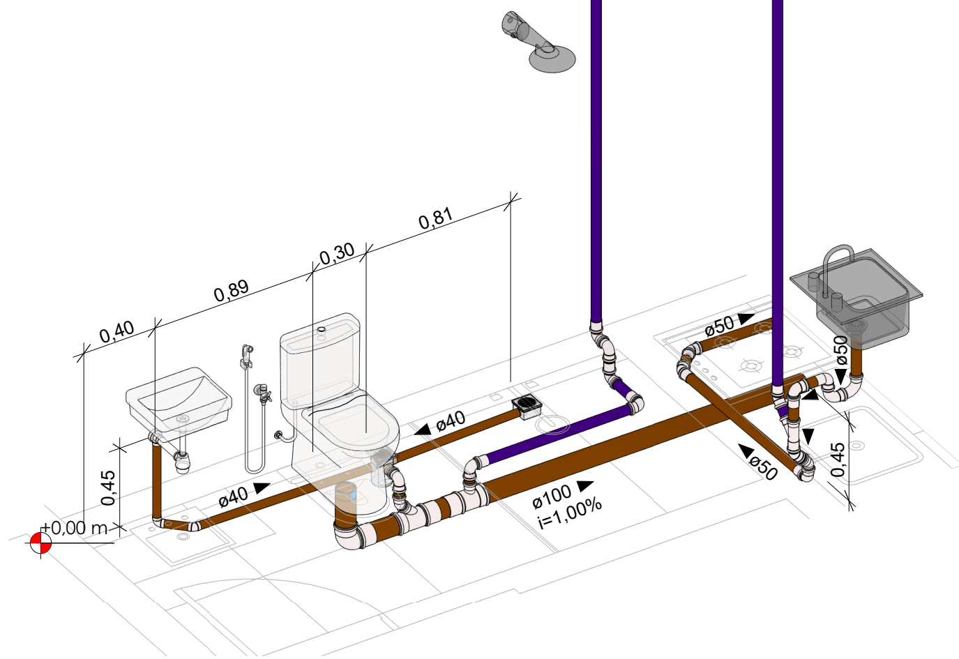
ISOMÉTRICAS 01 - WC_COPA - ESC 1/25
