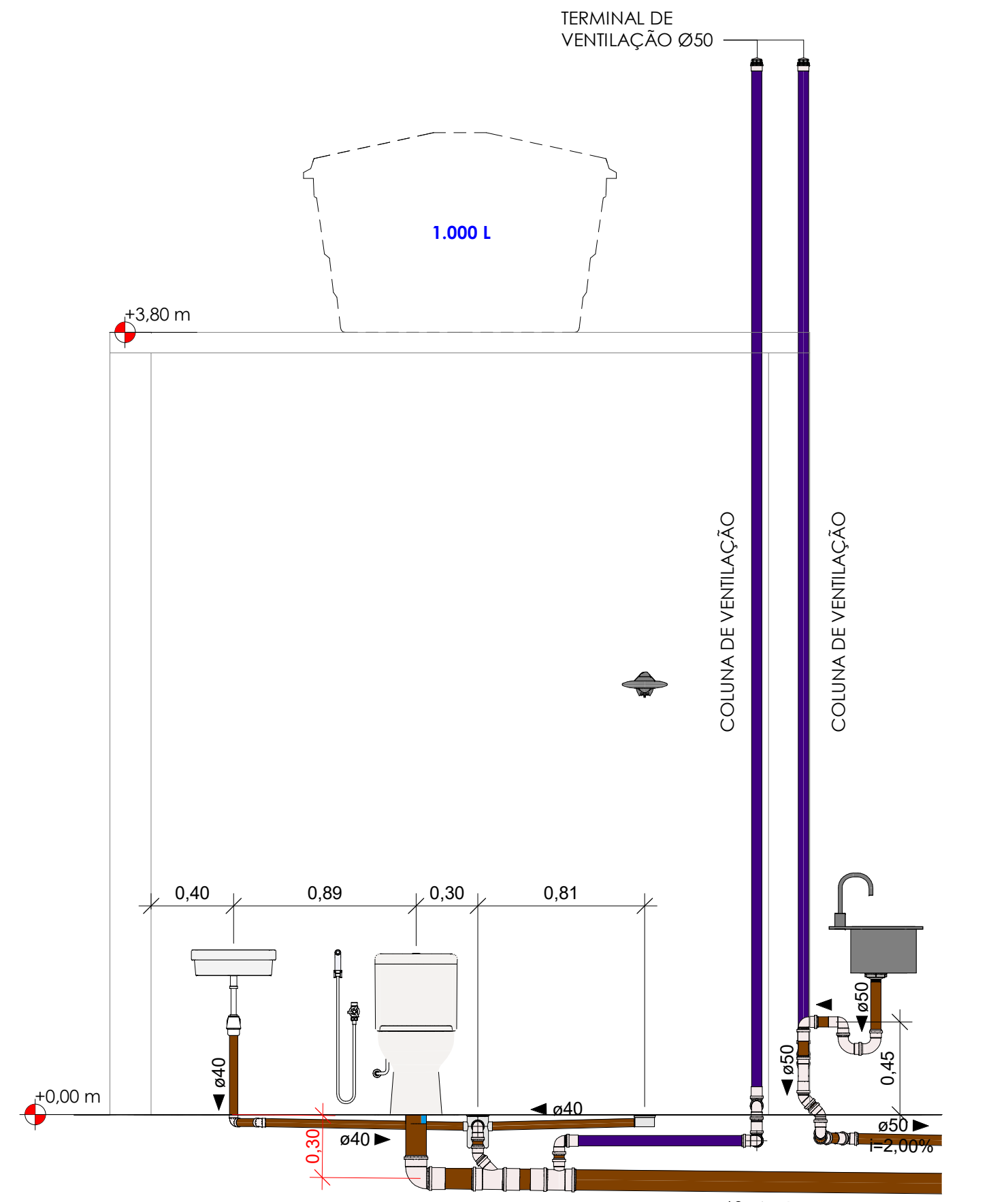
CORTE DD ESC 1/25
