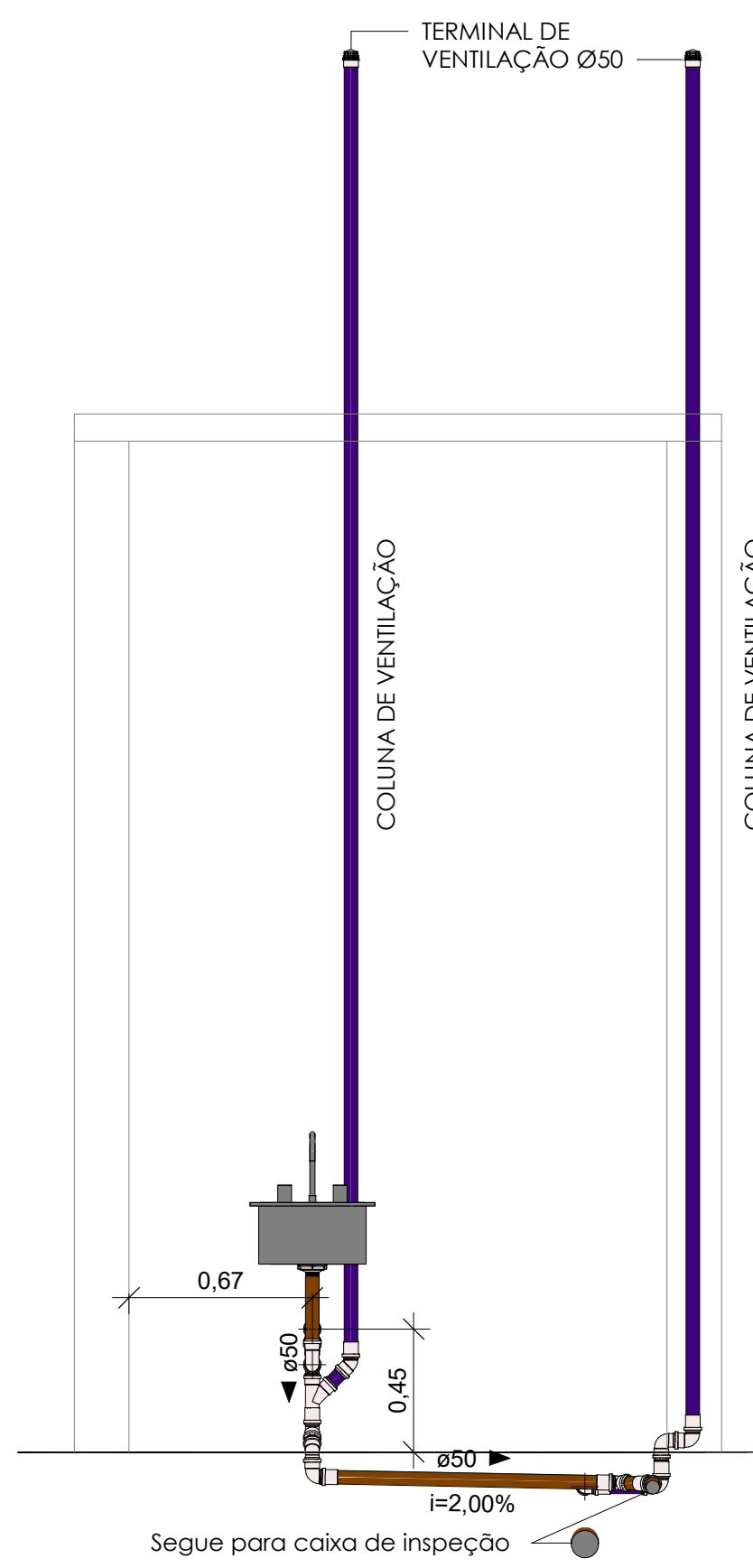
CORTE EE ESC 1/25
