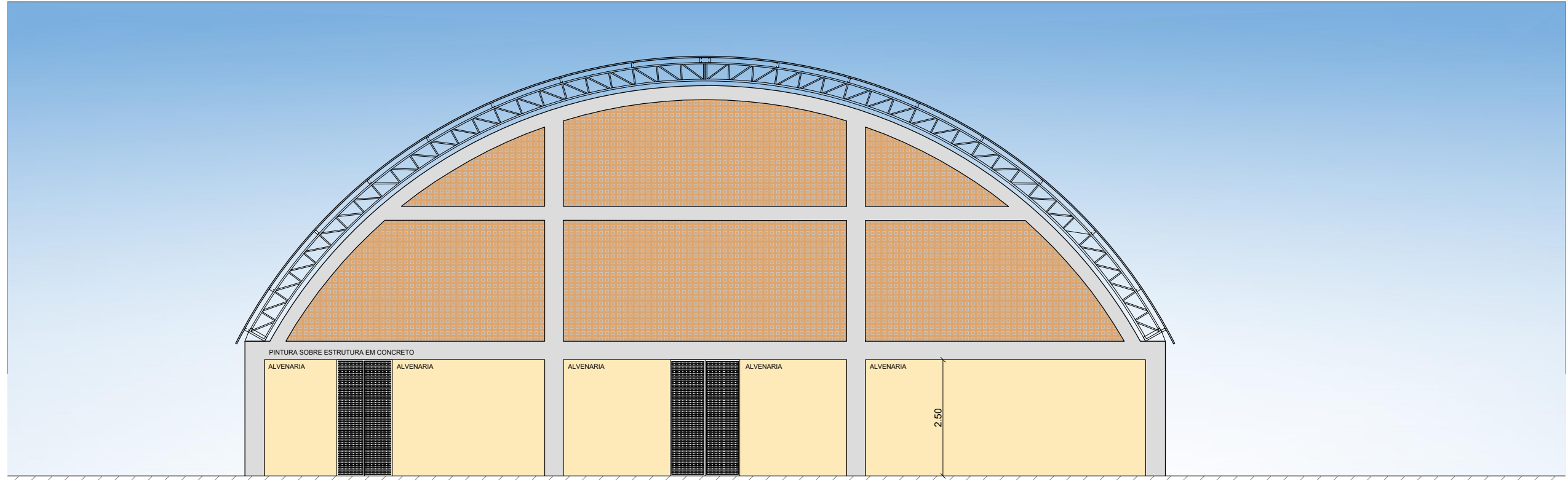
FACHADA 03 Escala 1:100
