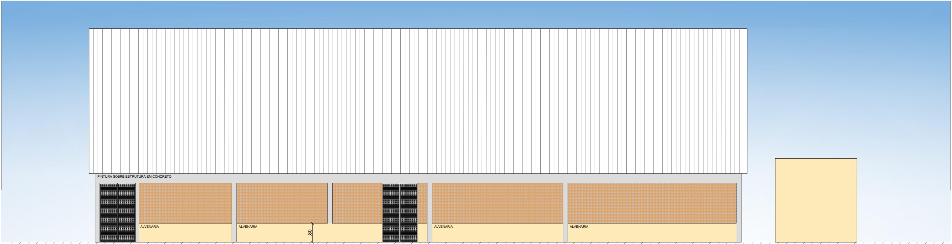
FACHADA 02 Escala 1:100
