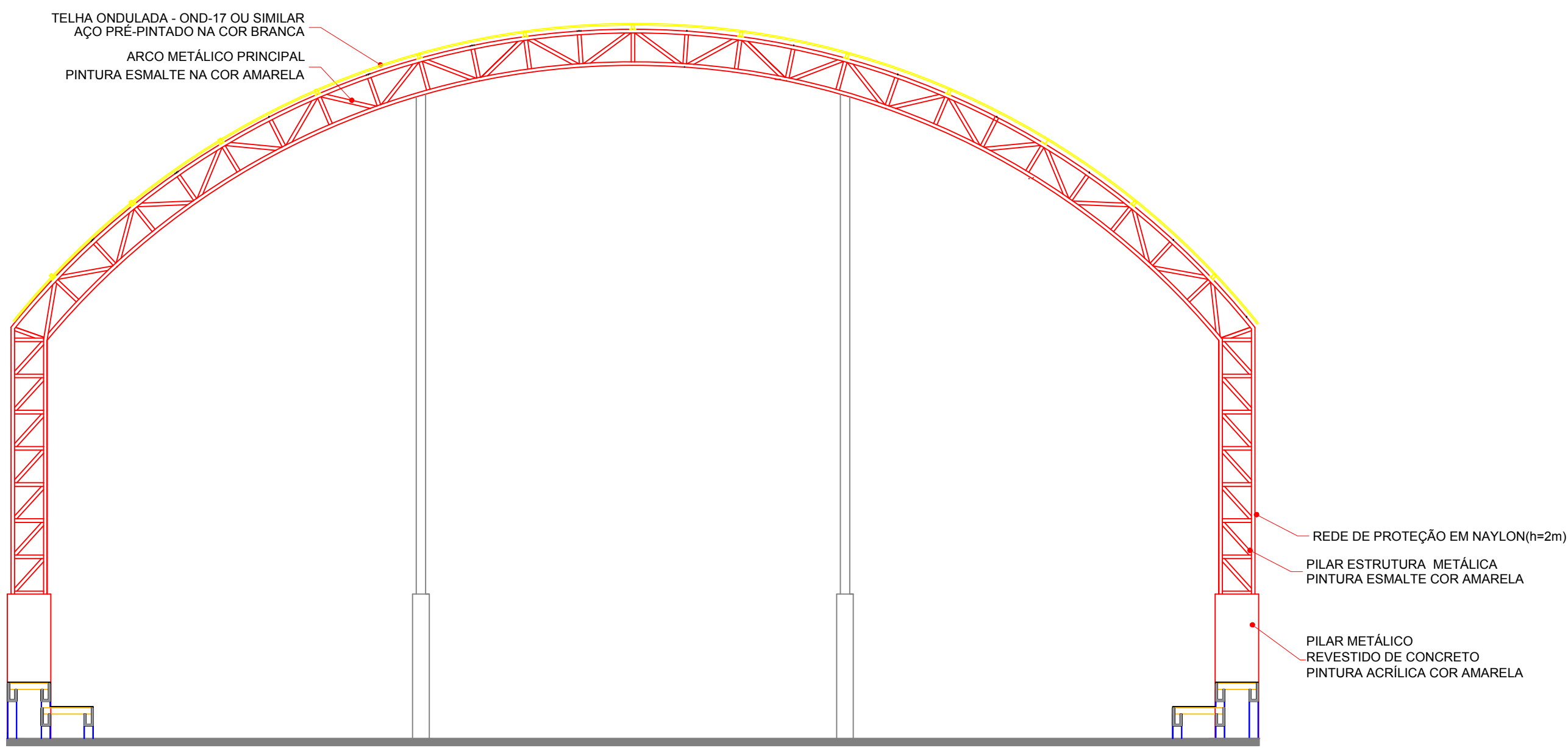
CORTE AA - QUADRA ESCALA 1:50
