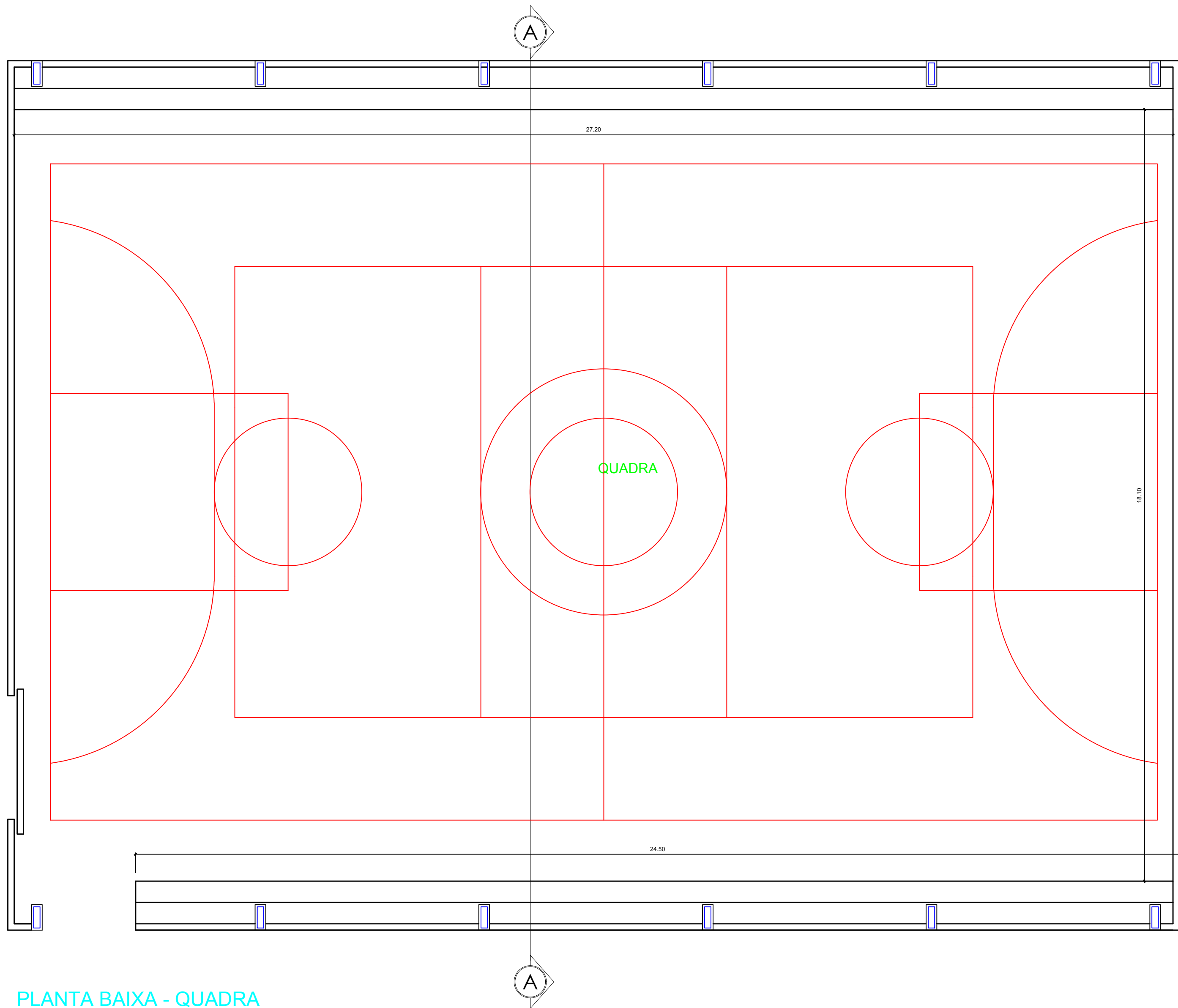
PLANTA BAIXA - QUADRA ESCALA 1:50
