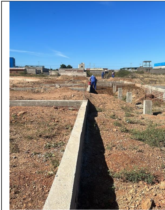
FOTO 1 – Execução de aterro compactado em camadas
