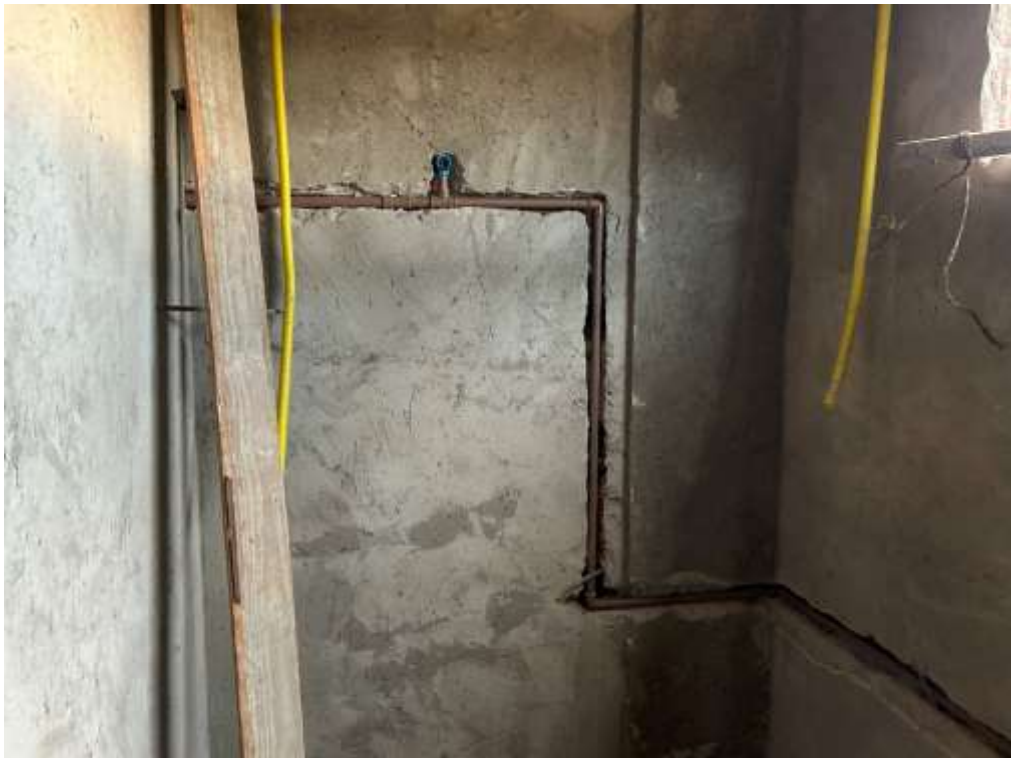
Figura 35: Execução das instalações hidrossanitárias.
