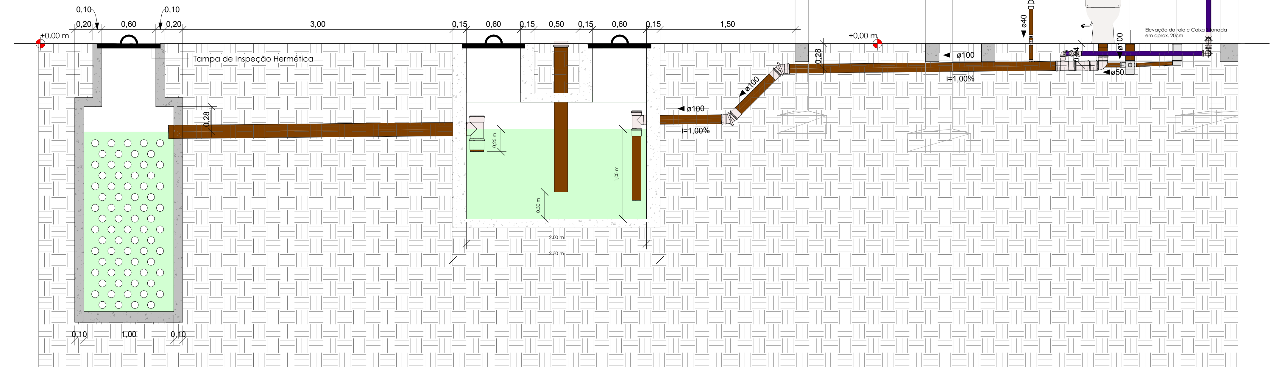
CORTE AA
