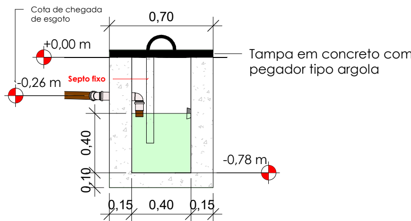
CORTE BB
