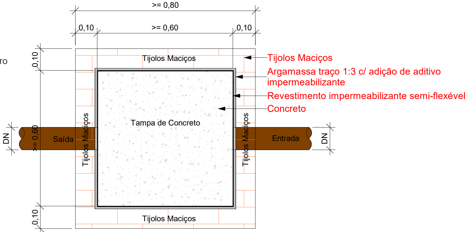
Planta Baixa - Caixa de inspeção 1 : 10
