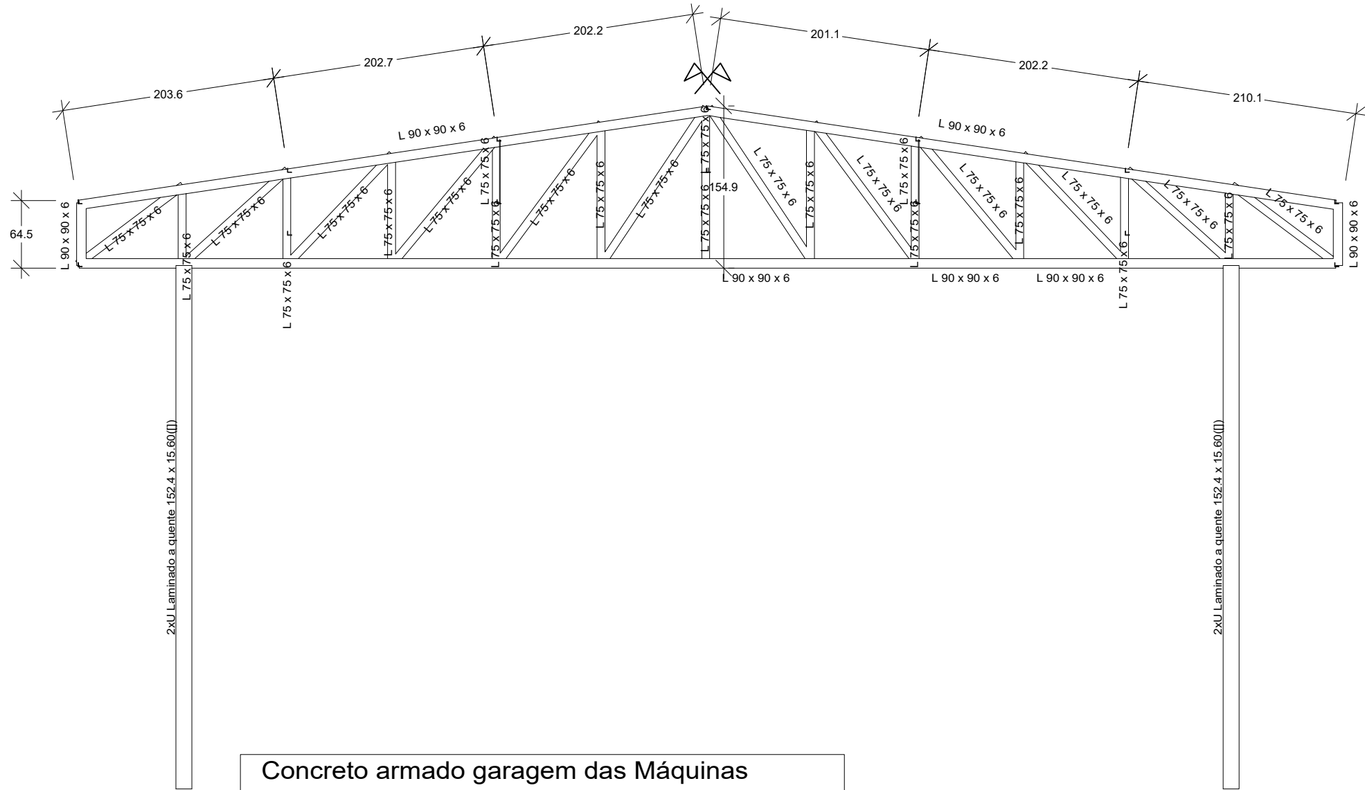
Estrutura 1: 2D: Pórtico Central
