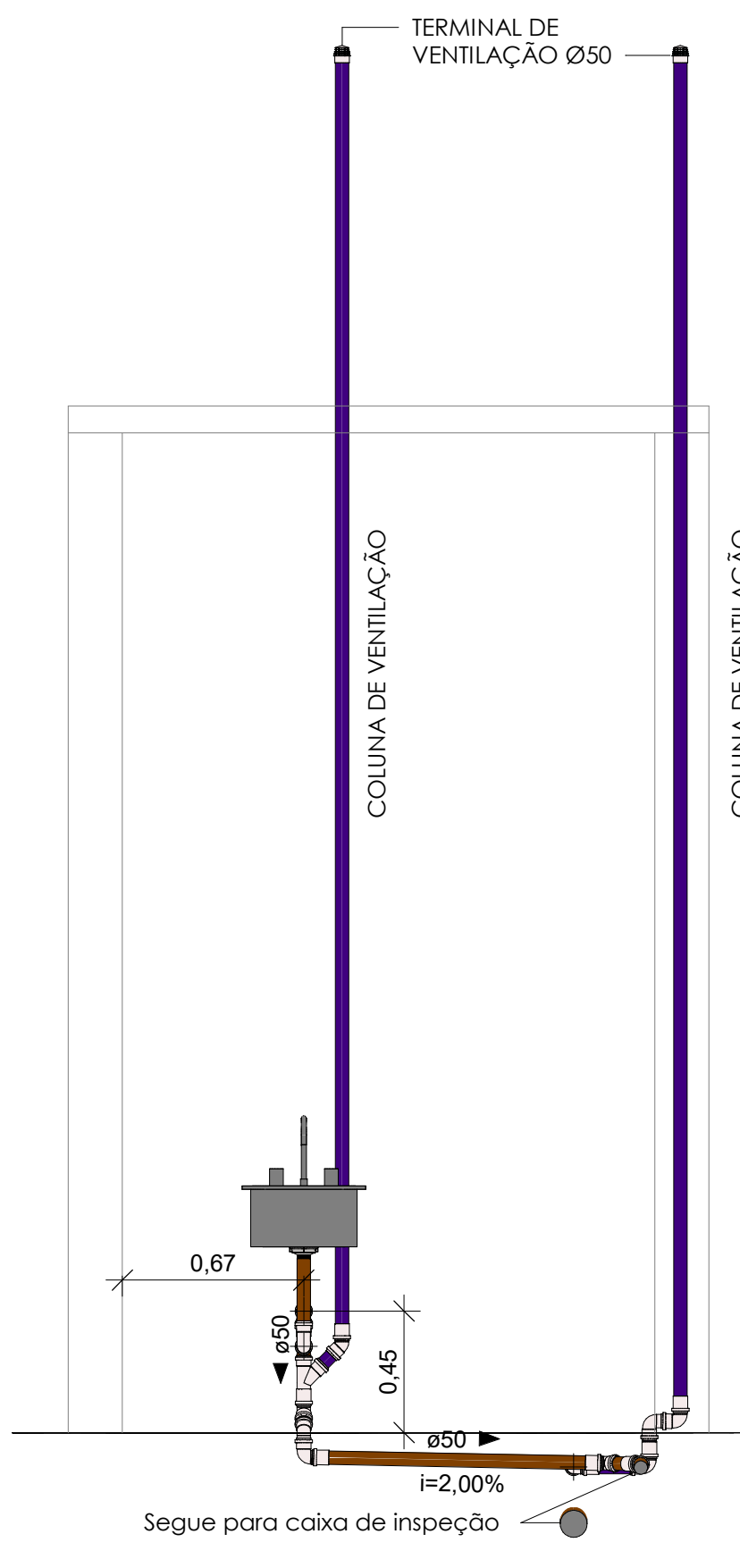
CORTE EE
