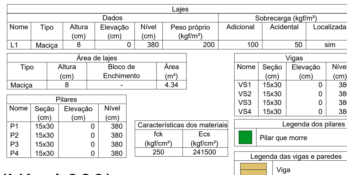
Forma do pavimento +380 (Nível 380) escala 1:50
