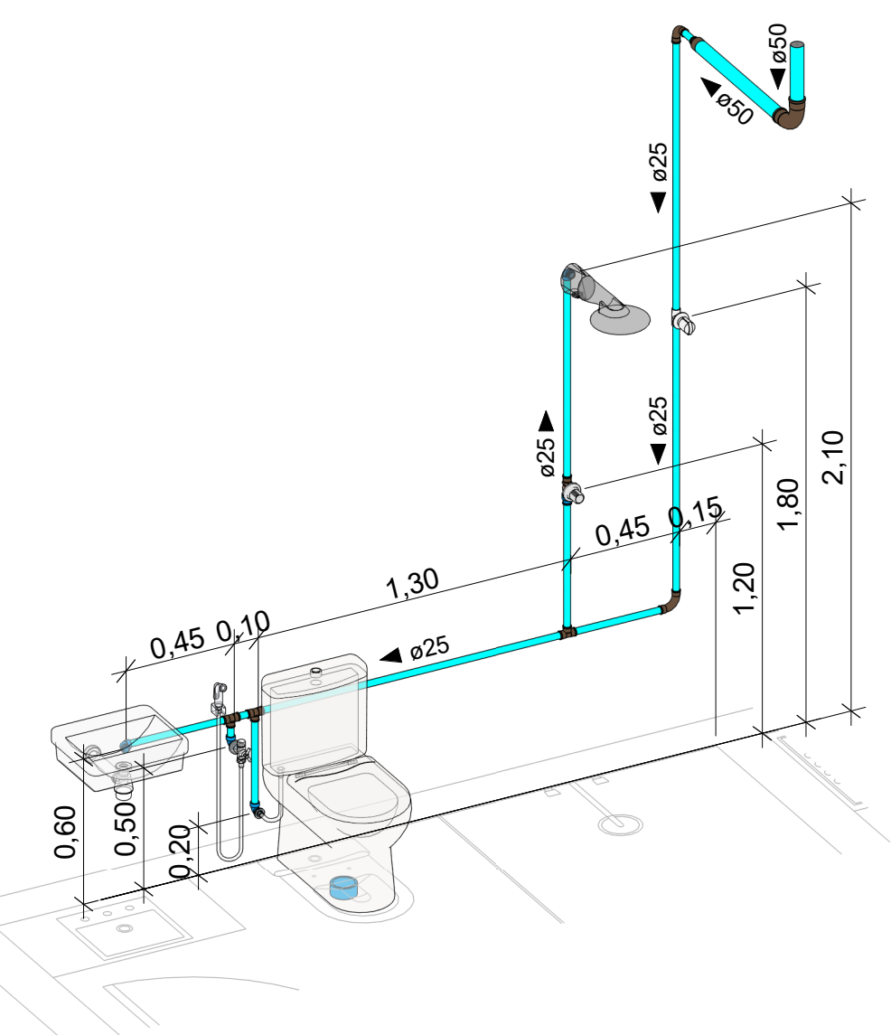
ISOMÉTRICA 03 - WC - ESC 1/25
