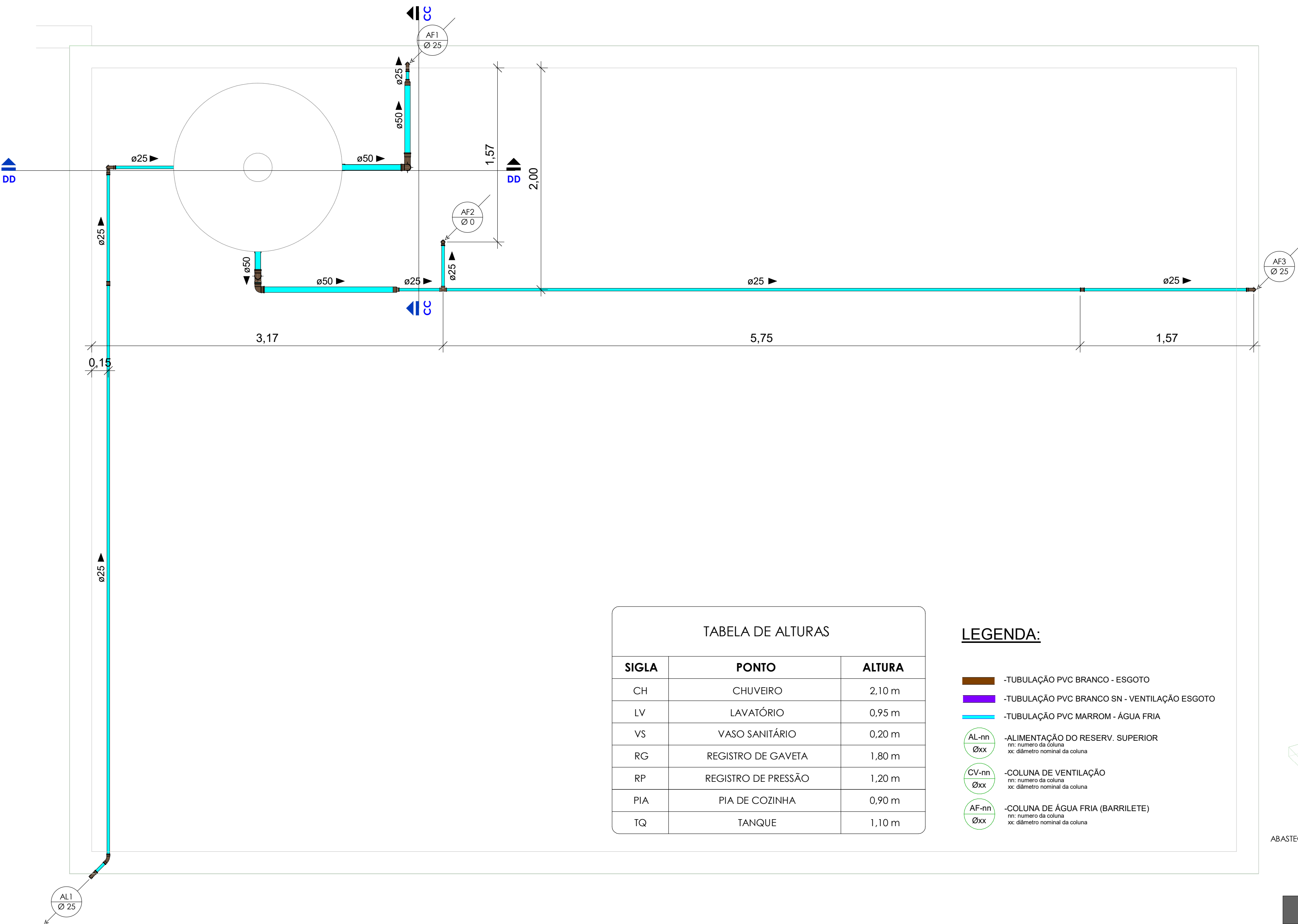
PLANTA BAIXA_CAIXA_D'ÁGUA_02 - ESC 1/25
