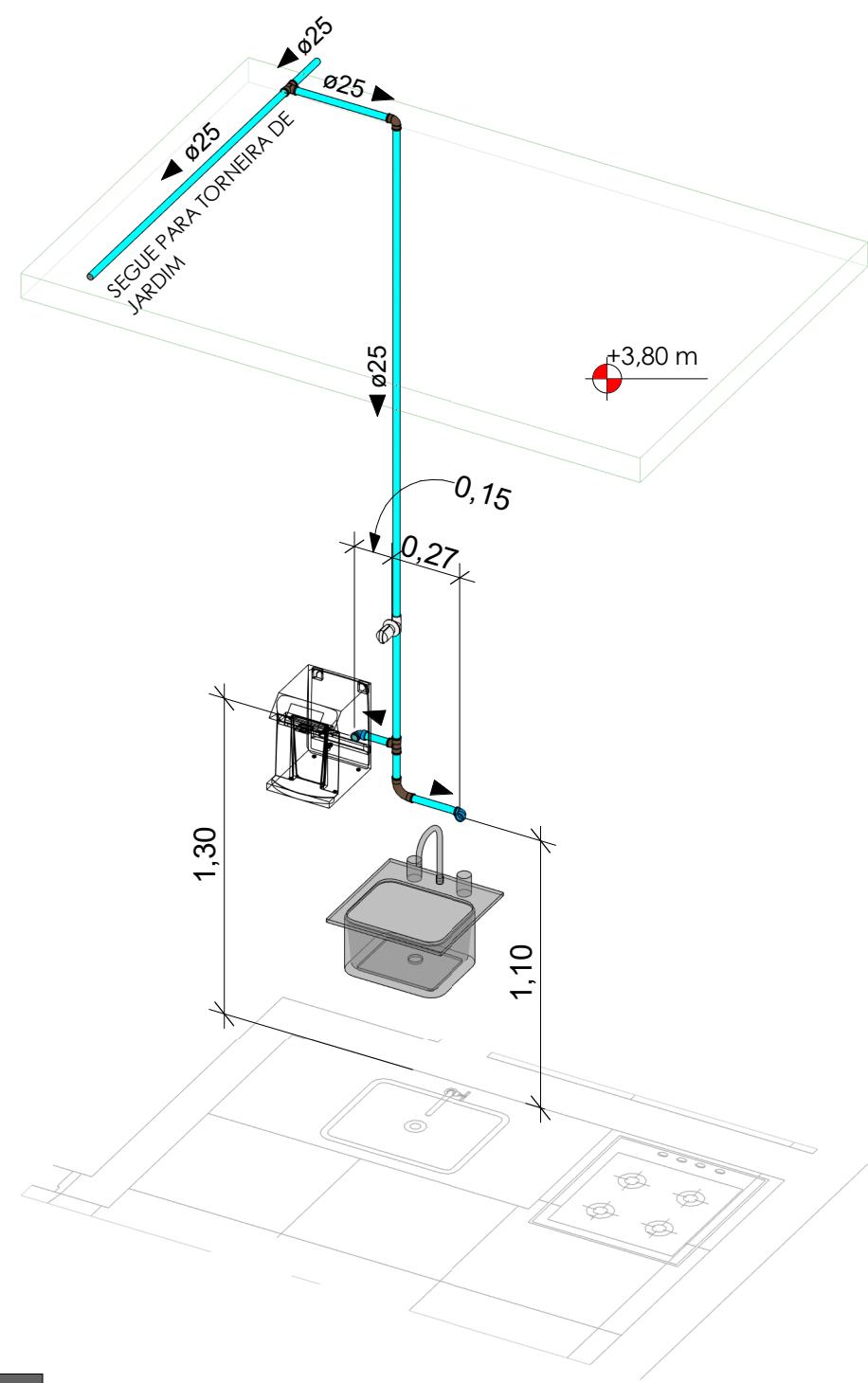
ISOMÉTRICA 04 - COPA - ESC 1/25
