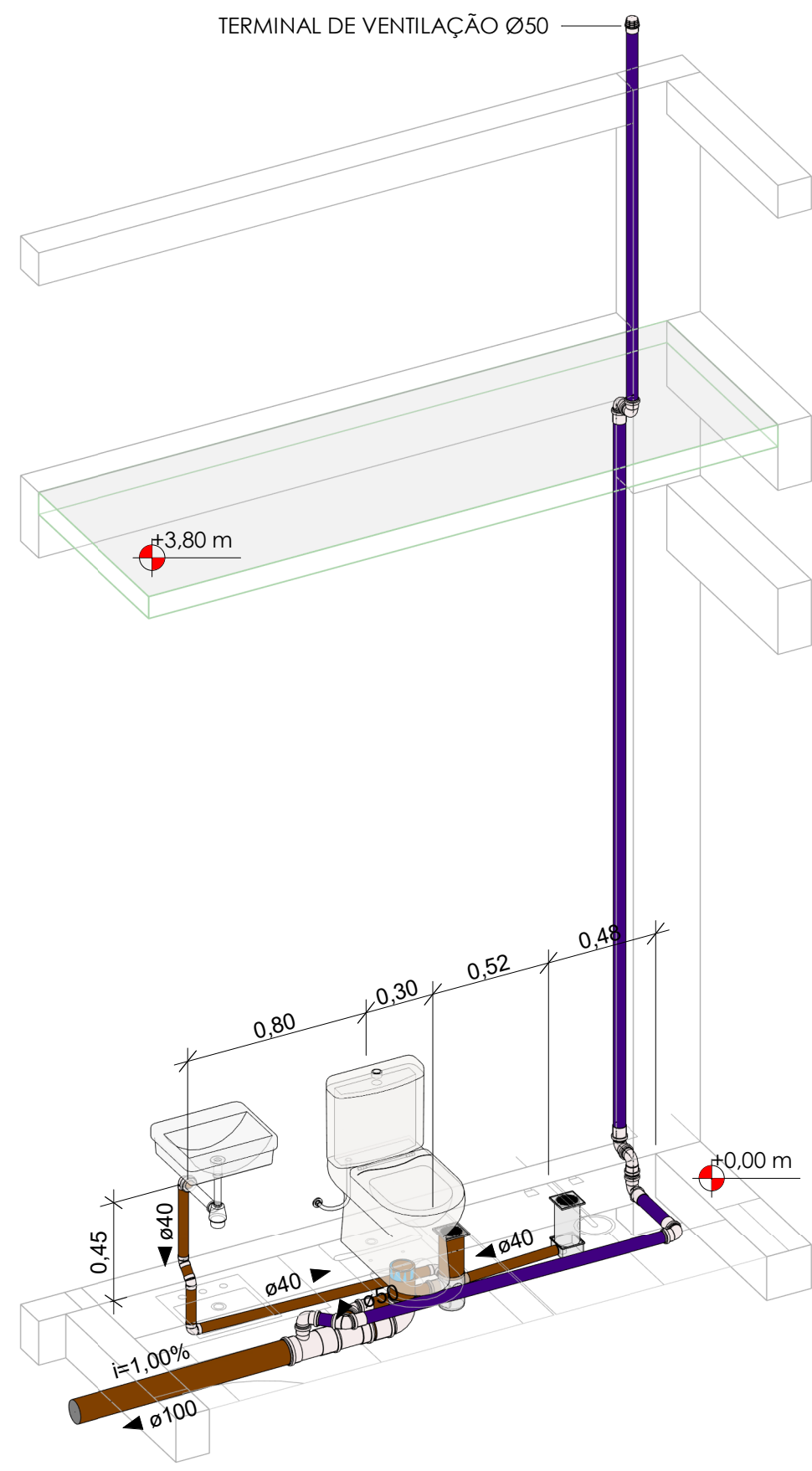
ISOMÉTRICA 02 - WC_MONITORAMENTO - ESC
