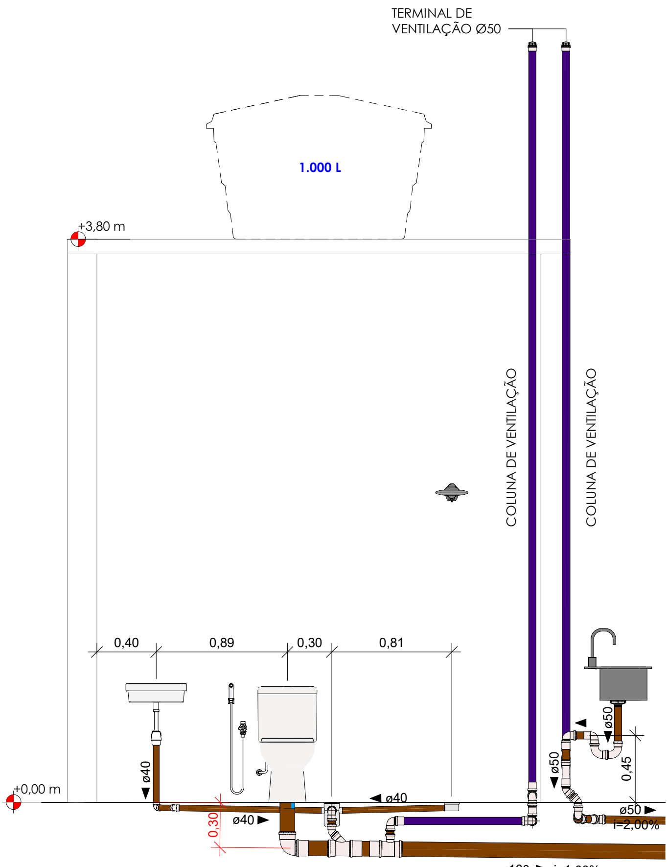
CORTE DD
