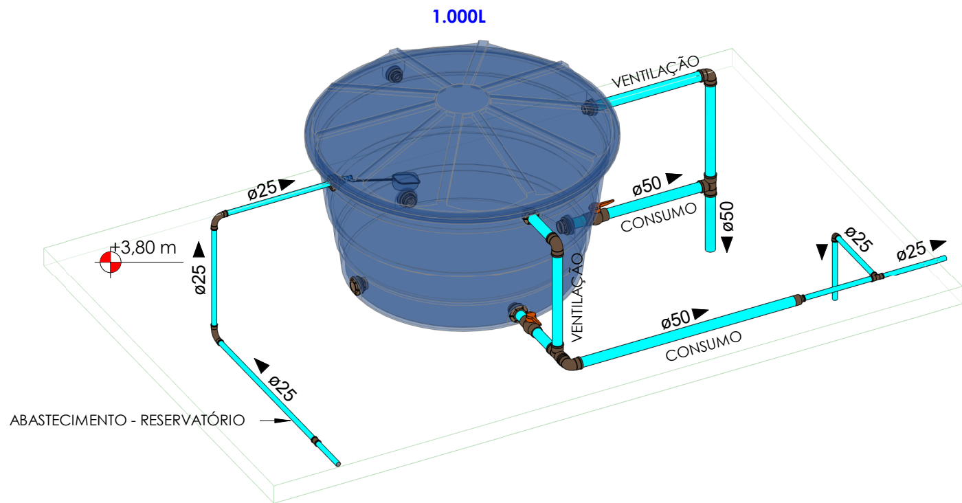
ISOMÉTRICA 05 - CAIXA D'ÁGUA - ESC 1/25
