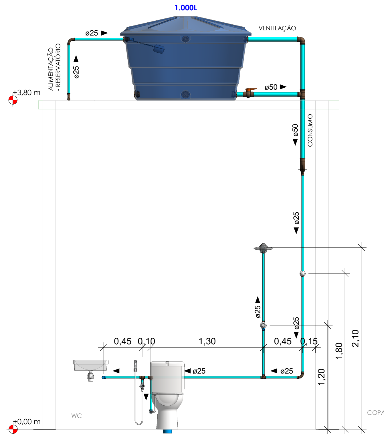
CORTE DD ESC 1/25
