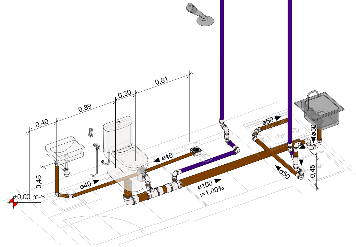
ISOMÉTRICAS 01 - WC_COPA - ESC
