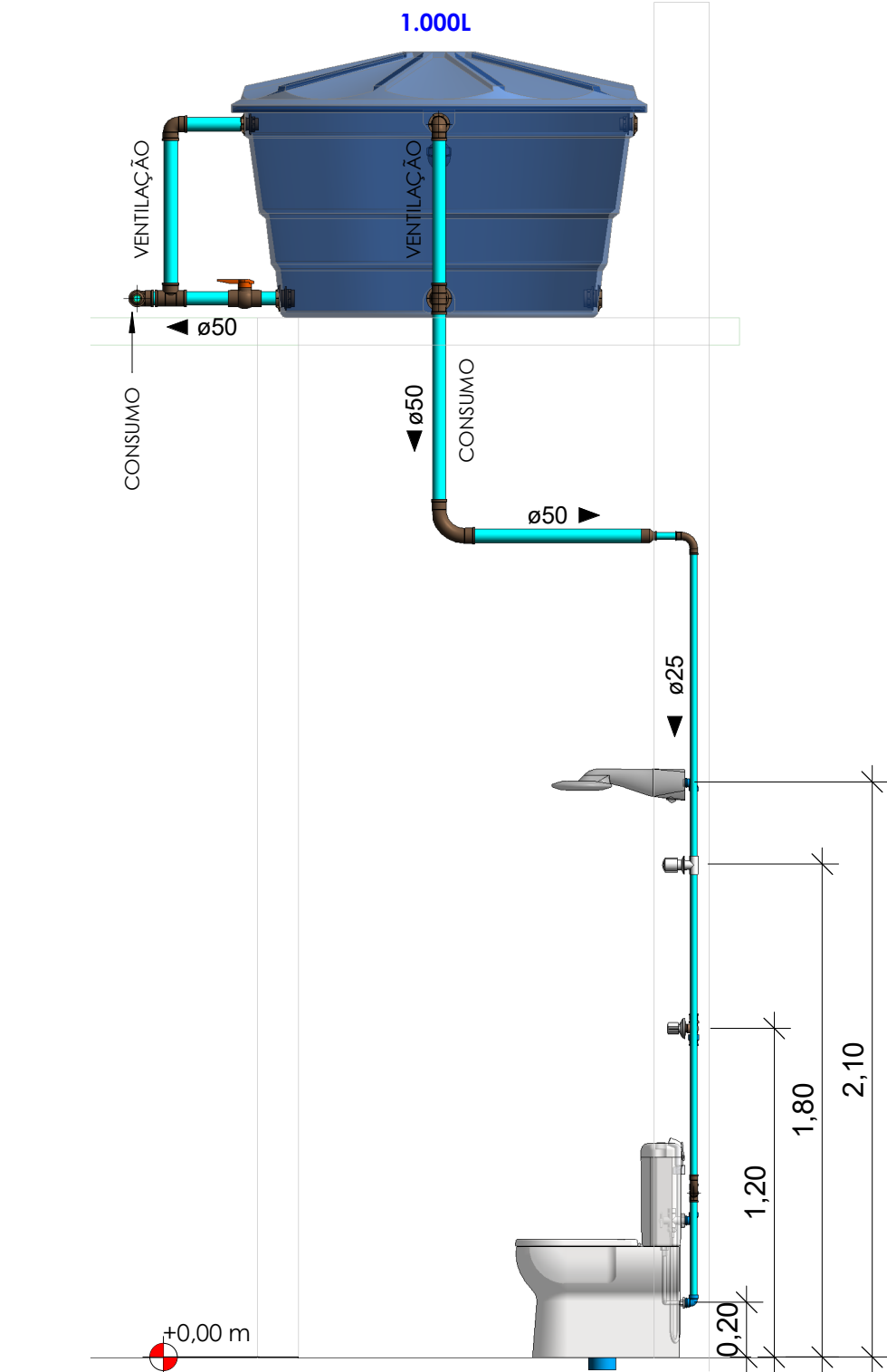
CORTE CC ESC 1/25
