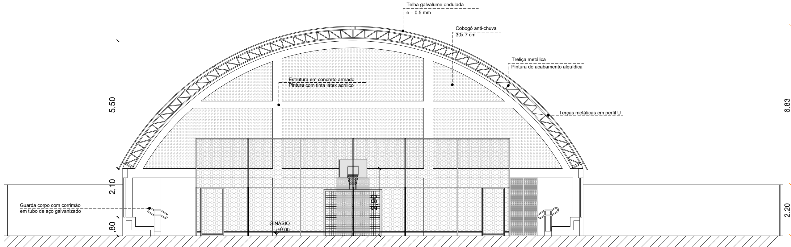
CORTE C-C escala 1/100
