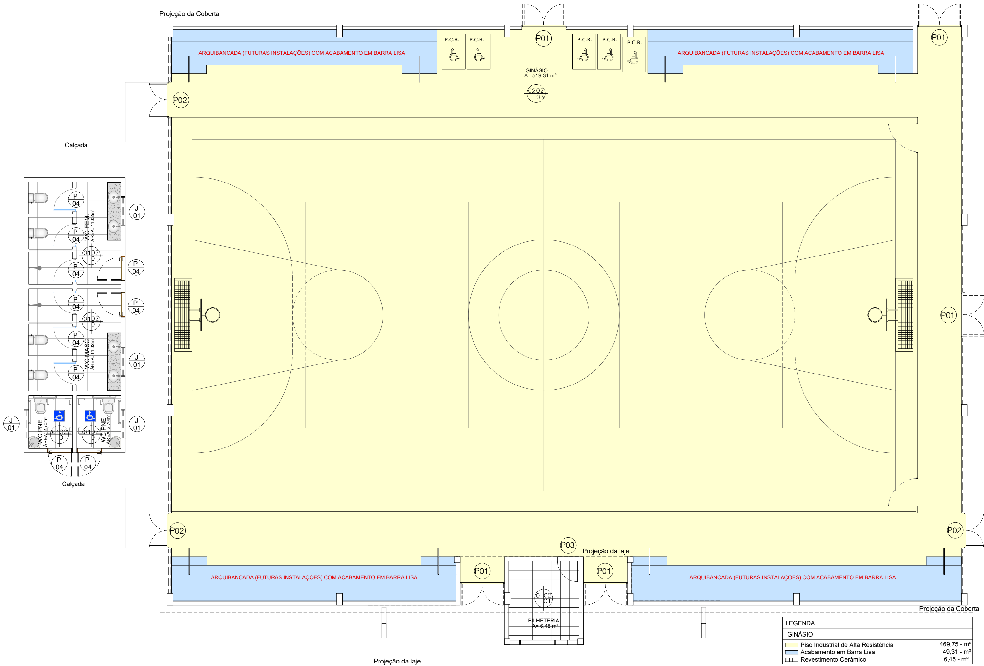
PLANTA BAIXA - ACABAMENTOS E ESQUADRIAS ESC.: 1:100
