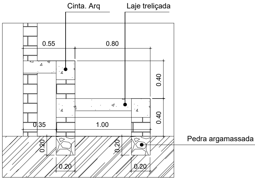
Corte - Arquibancada ESC.: 1:25
