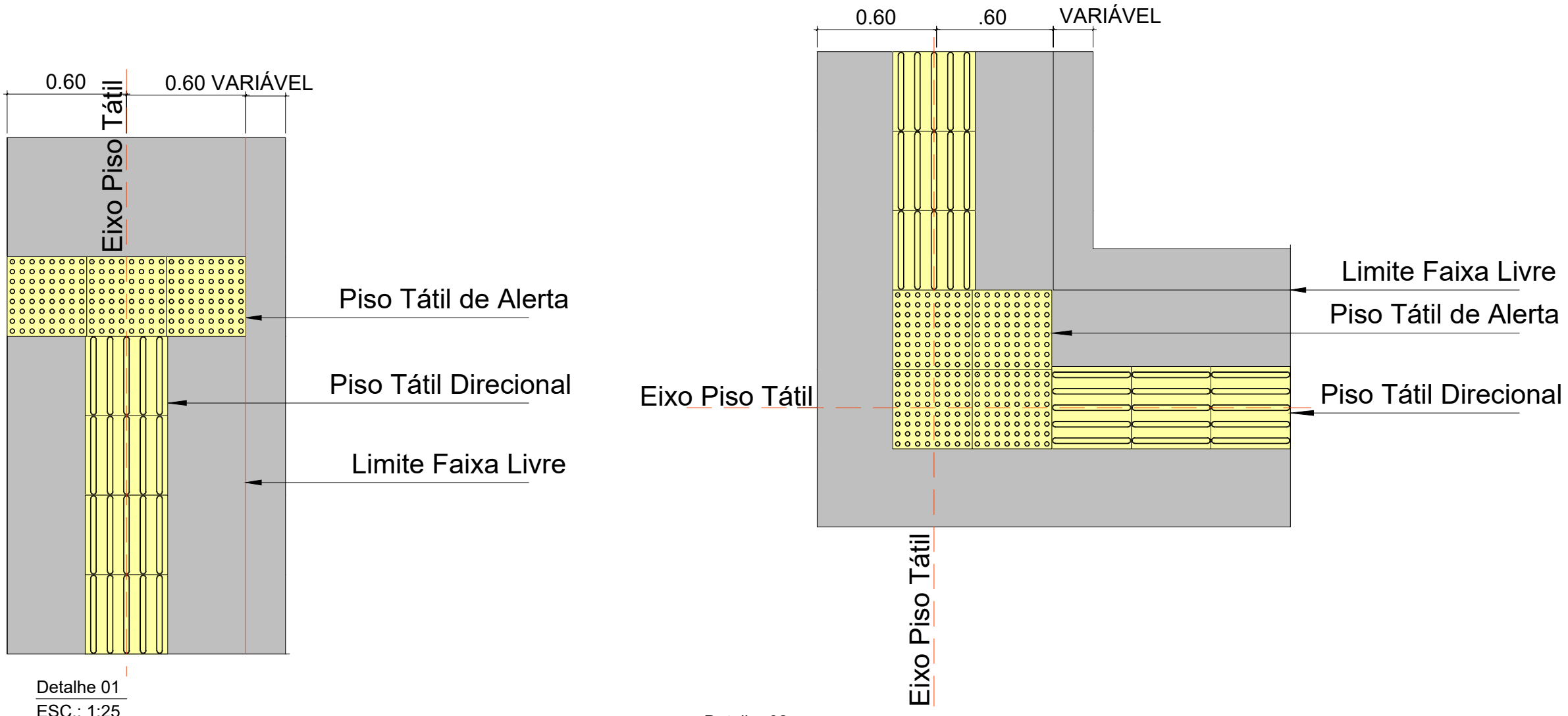
Detalhe 02 ESC.: 1:25
