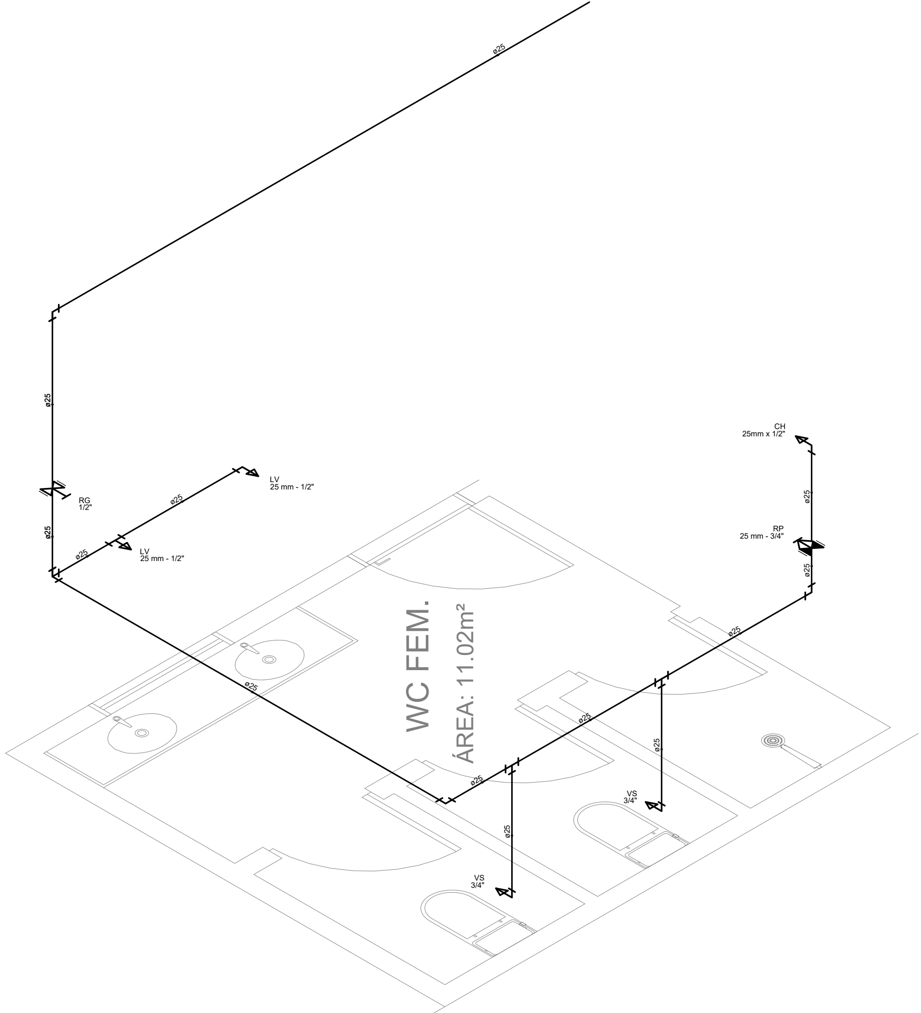
Detalhe H3 Escala 1:25
