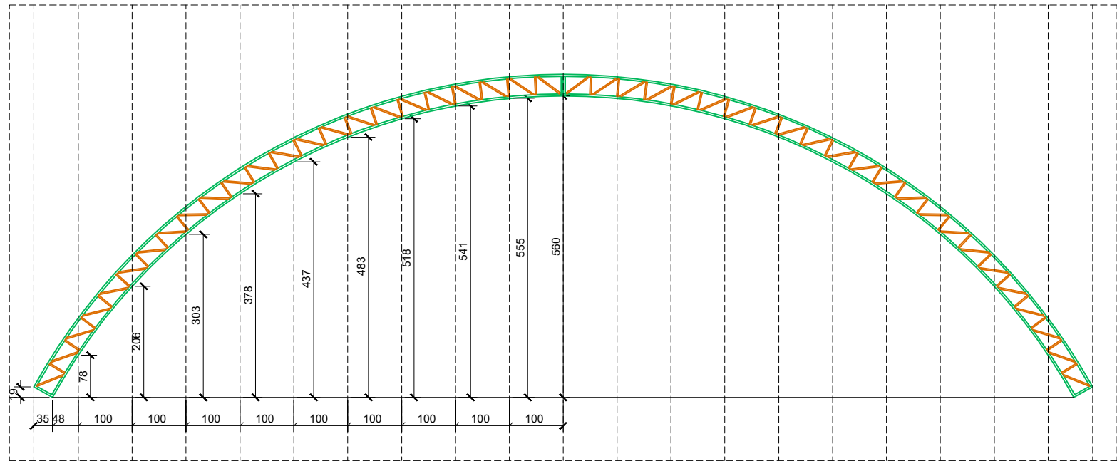
DETALHE DE FABRICAÇÃO DO ARCO (6x)
