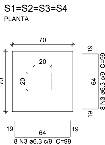
Detalhe Fundação – Caldeira escala 1/20
