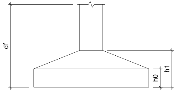
Detalhe estrutural – Caldeira escala 1/50
