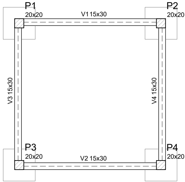
Forma Baldrame – Caldeira escala 1/50
