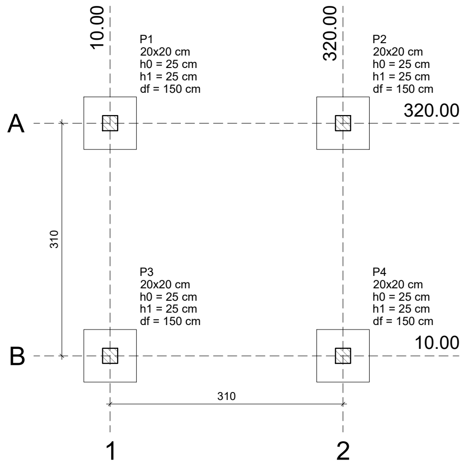
Localização estrutural – Caldeira escala 1/50
