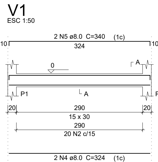
Detalhe Fundação – Vigas escala 1/50
